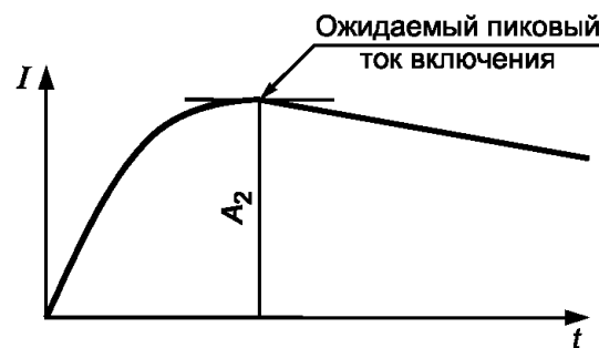
Рисунок 7б — Калибровка испытательной цепи для постоянного тока
