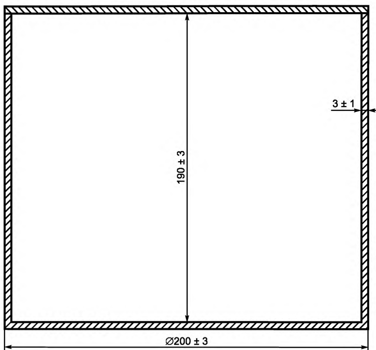
Рисунок 1 — Геометрия проекций
