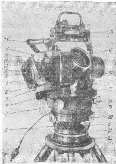
Рис. 10.16. Теодолит ДКМ3-А. Вид со стороны контактного микрометра:
