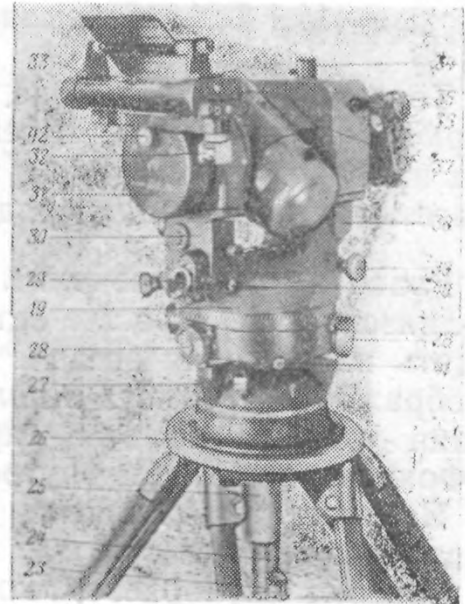
Рис. 10.16. Теодолит ДКМ3-А. Вид со стороны контактного микрометра:
