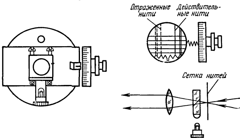
Рис. 10.49. Микрометр с автоколлимационным окуляром
