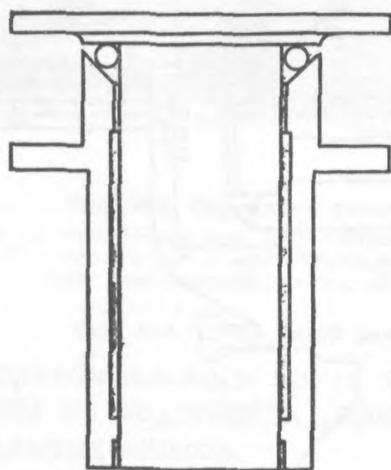
Рис. 10.13. Кинематическая схема вертикальной оси теодолита Т4
