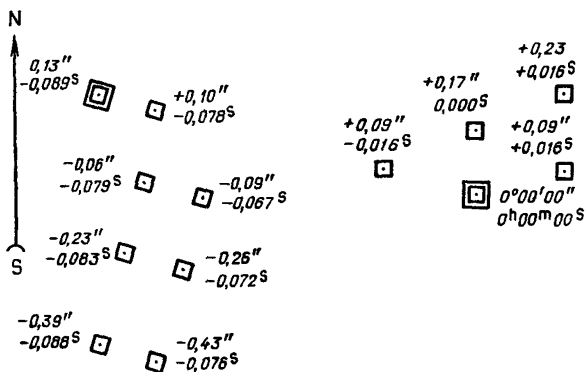
Рис. 3.3. Схема расположения столбов (Ташкент)
