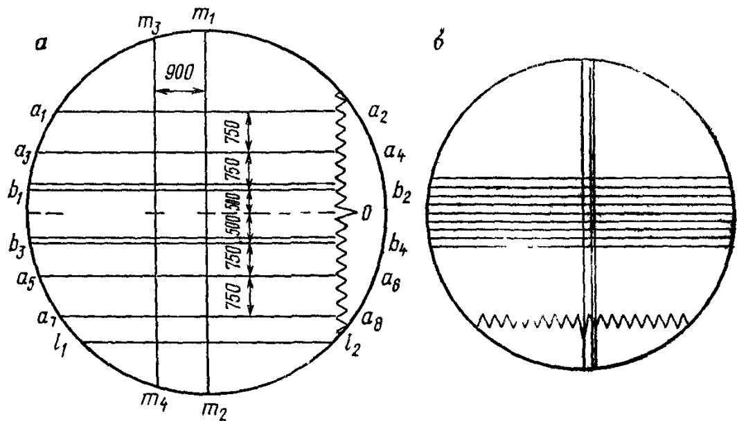
Рис. 10.4. Сетки нитей АУ 2/10:
