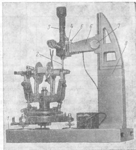
Рис. 10.40. Прибор для исследования цапф контактным способом
