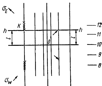
Рис. 35. Сетка нитей микрометров теодолитов Вильд Т4 и ДКМЗ-А
