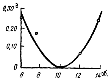
Рис. 11.7. График поправок за годовые погрешности винта микрометра
