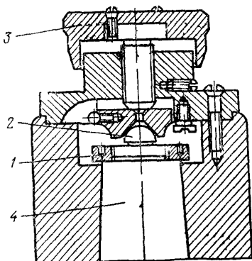
Рис. 105. Регулировочный конец вертикальной оси АУ 2/10 1 — ограничительная гайка, 2 — шаровая опора, 3 — регулировочный грибок, 4 — вертикальная ось
