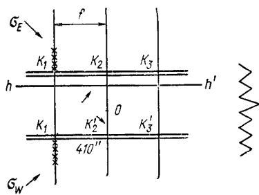
Рис. 34. Сетка нитей контактного микрометра геодалита АУ 2/10
