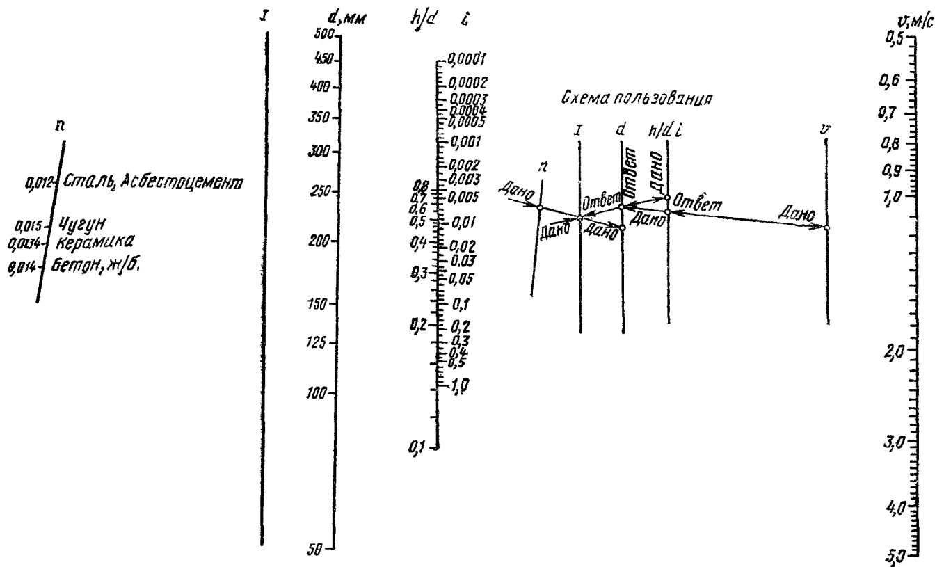
Рис. 1. Номограмма для определения гидравлического уклона канализационных трубопроводов
