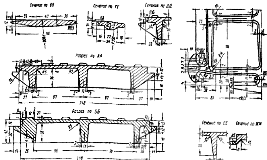
Рис. 2. Плита чугунная с опорными выступами для полов, укладываемая на песке Детали
