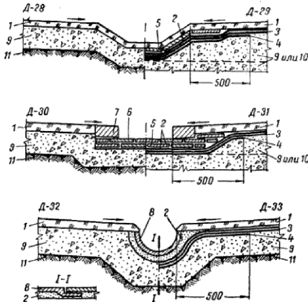
Рис. 6. Сточные лотки
