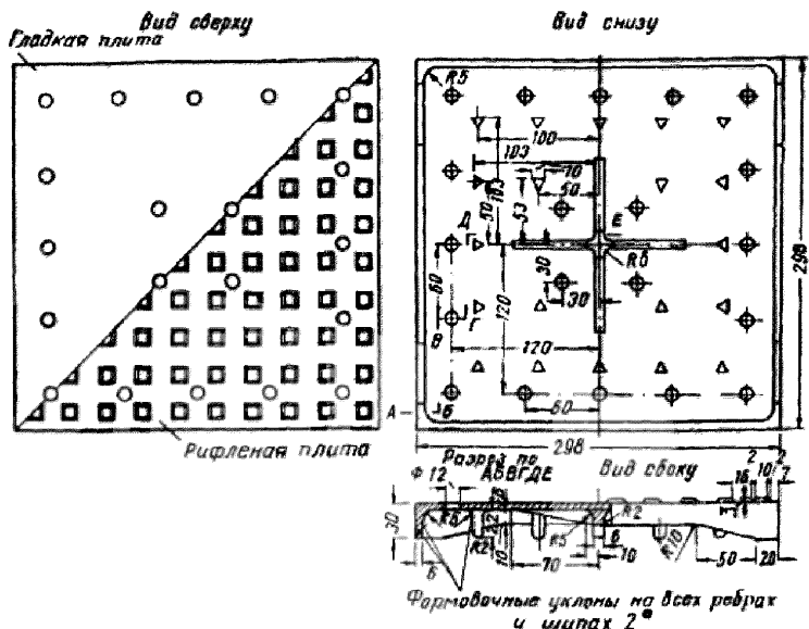
Плита чугунная дырчатая с шпалами для полов, укладываемая на растворе. Вес плиты: гладкой — 4,5 кг, рифленой — 4,8 кг
