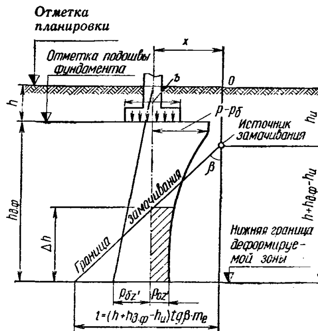
Рис. 4. Схема для расчета ограниченной величины \Delta h замачивания нижней зоны основания под вертикальной осью фундамента в случае, если она находится в стороне от источника замачивания
