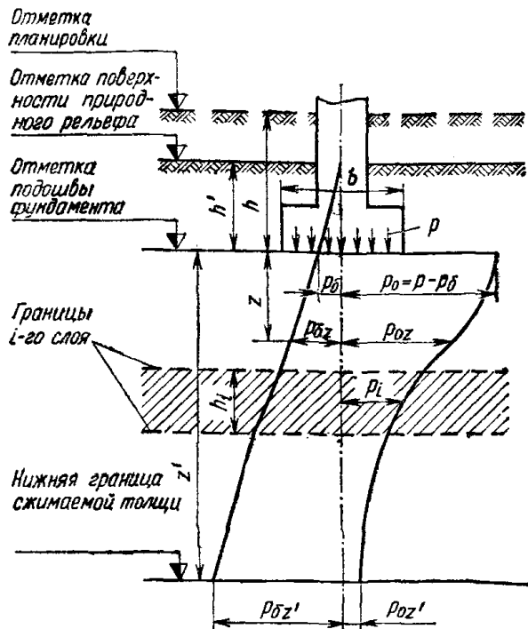
Рис. 1. Схема для расчета осадок методом послойного суммирования
