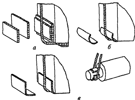
Рис. 33. Строповка грузов с использованием деревянных проставок (а), проставок из разрезанной трубы (б), проставок из резиноканевых шлангов, плоских ремней (е)
