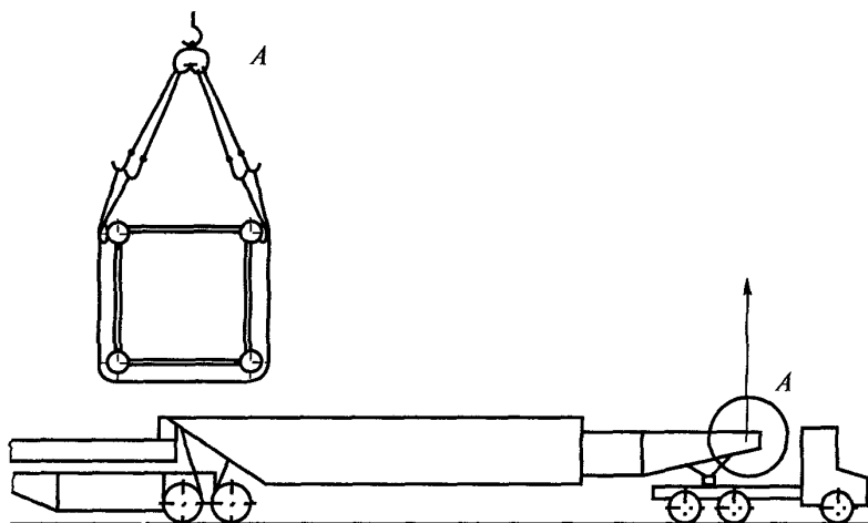
Схема 3. Строровка башни крана за оголовок при снятии крана с тягача
