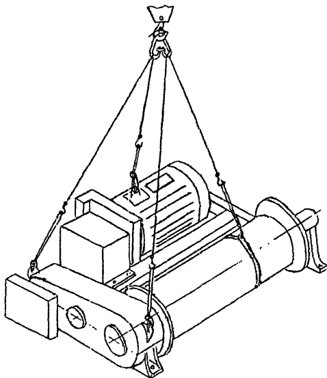
Схема 7. Стрповка грузовой лебедки
