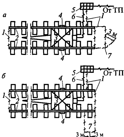
Рис. 12. Схемы заземления пути:
