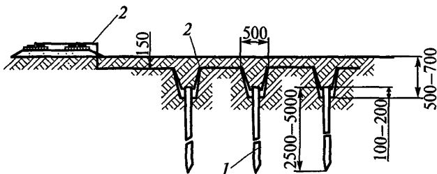
Рис. 13. Схема соединения вертикальных заземлителей:
