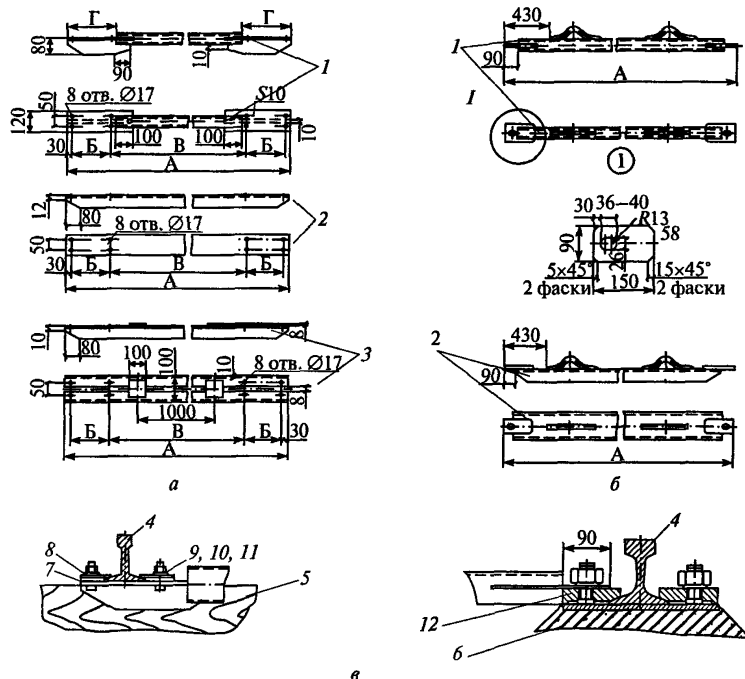
Рис. 9. Конструкции стяжек:
