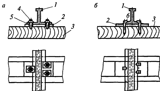
Рис. 6. Крепление рельса к полушпале:
