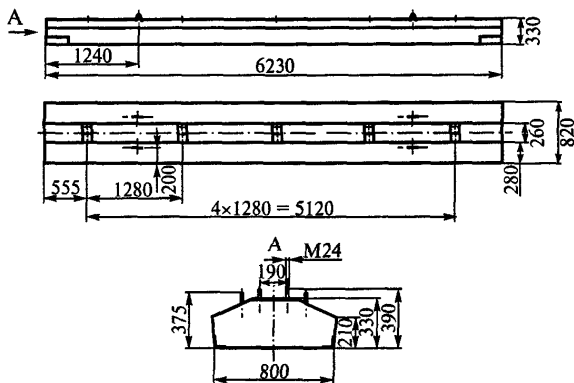
Рис. 2. Железобетонная балка типа БРП-62.8.3
