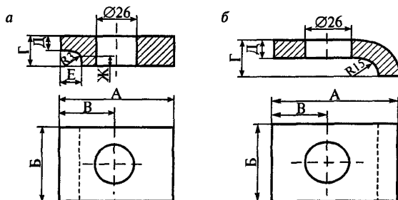
Рис. 7. Прижим:
