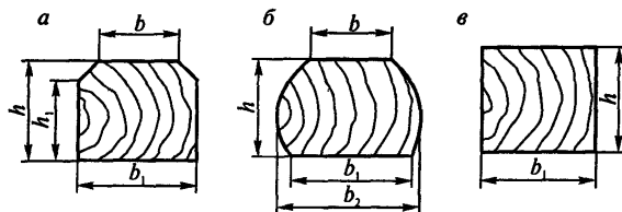
Рис. 3. Поперечное сечение деревянных полушпал:
