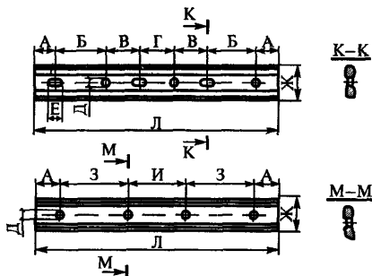
Рис. 8. Накладки двухголовые:
