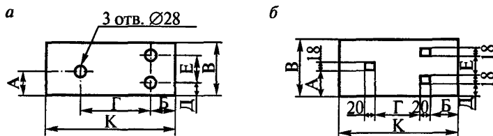
Рис. 5. Подкладки рельсов с креплением:
