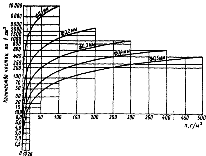
Рис.3. Логарифмические кривые зависимости количества частиц, приходящихся на 1 см 2 опыливаемой площади, от нормы расхода (г/м 2 ) для различных диаметров распыливаемых частиц.
