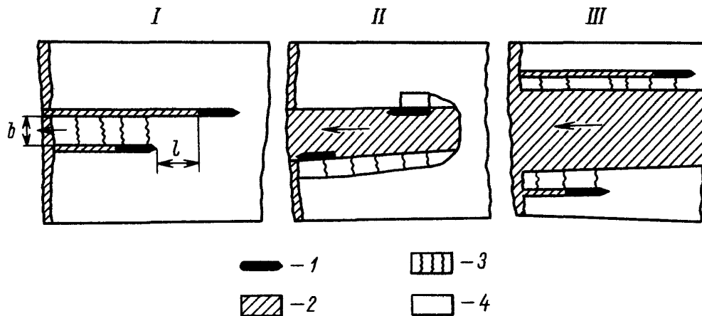
Рис.4. Порядок производства работ по образованию канала во льду с целью предупреждения весенних заторов льда
