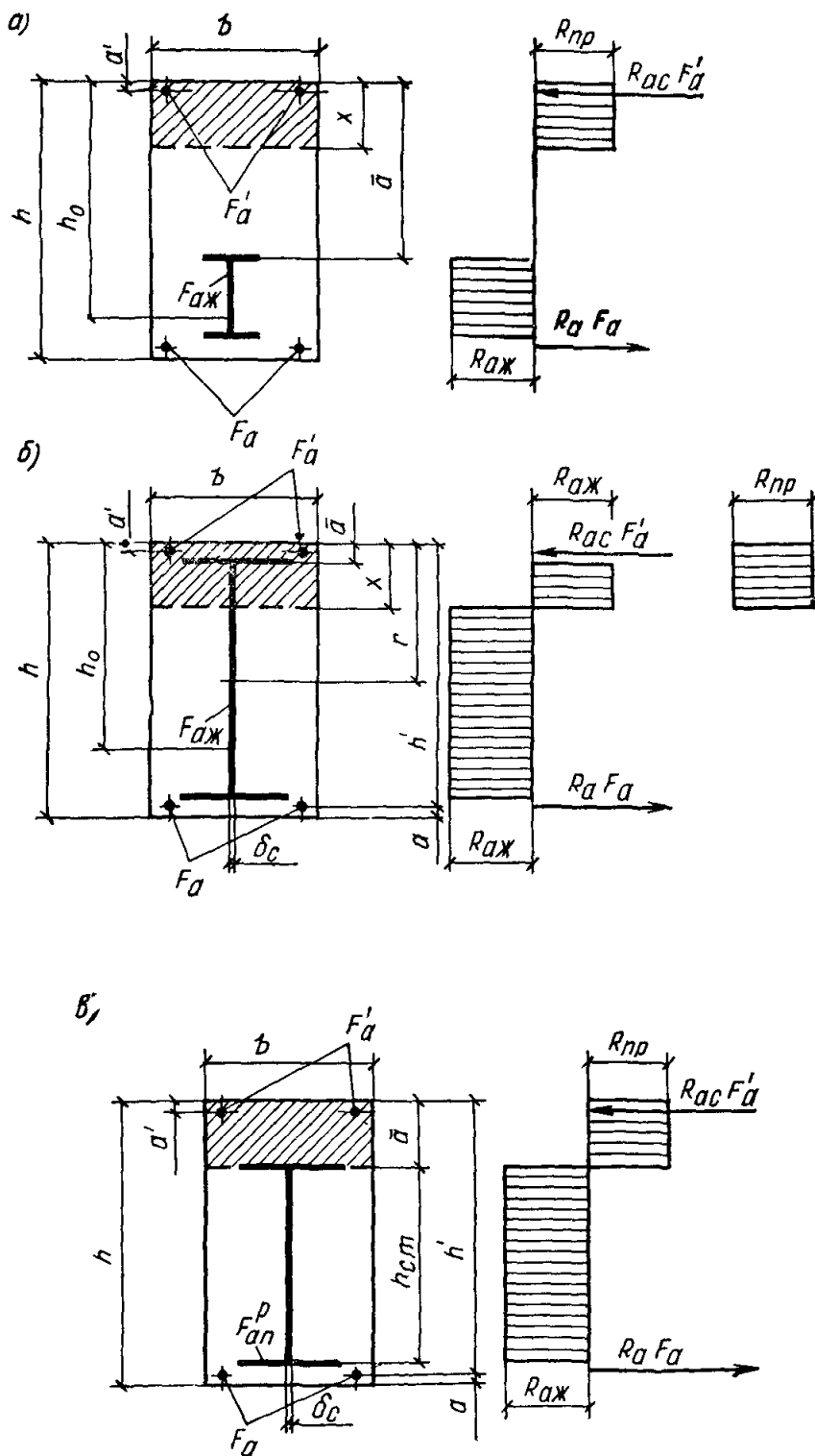
Рис. 1. Случай расположения нейтральной оси для прямоугольного сечения а — случай 1, б — случай 2, в — случай 3
