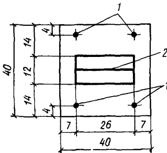
Рис. 18. К примеру расчета 8 1 — продольная арматура 2Ø32 А-III; 2 — стальной сердечник
