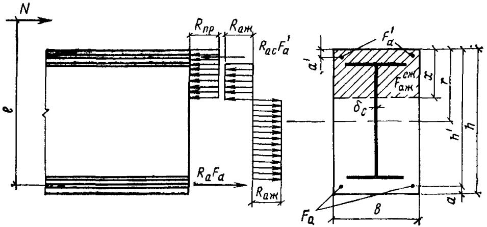
Рис. 13. Схема усилий в прямоугольном сечении сжатого элемента с жесткой арматурой в виде симметричного профиля, стенка которого расположена параллельно плоскости действия изгибающего момента
