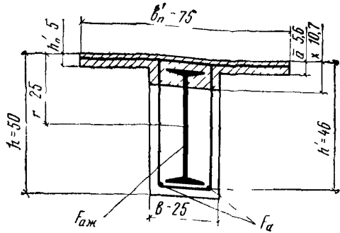
Рис. 7. К примеру расчета 5
