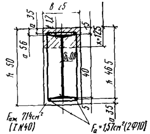
Рис 4 К примеру расчета 2
