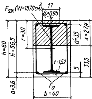
Рис. 19. К примерам расчета 9 и 10
