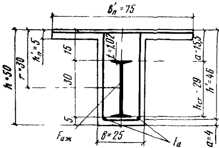
Рис. 8. К примеру расчета 6
