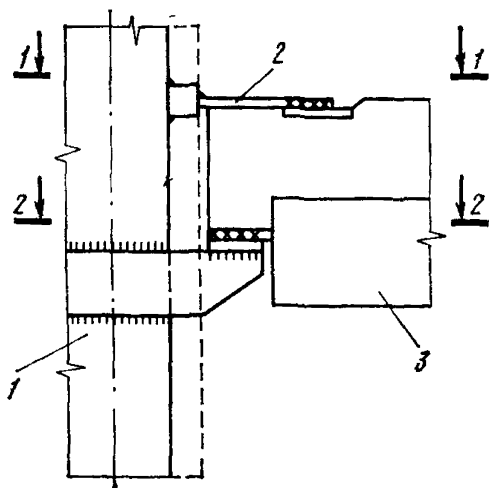
Рис. 22. Стык ригеля с железобетонной колонной с жесткой арматурой
