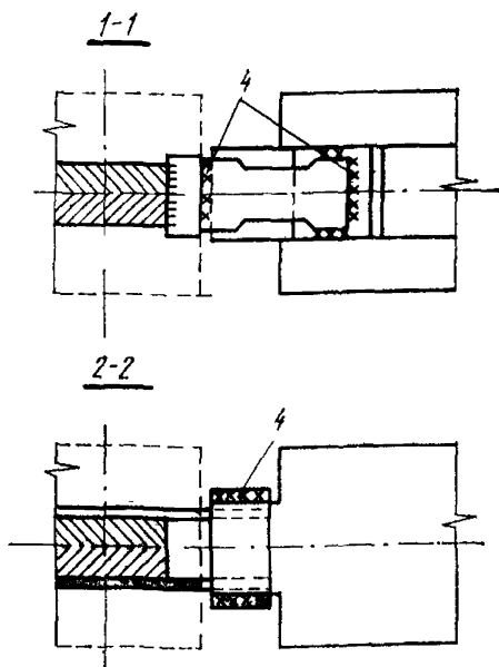
Рис. 22. Стык ригеля с железобетонной колонной с жесткой арматурой
