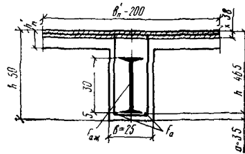
Рис. 6. К примеру расчета 4
