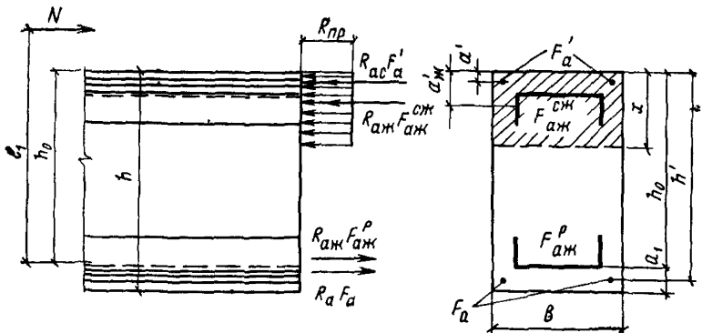
Рис. 11. Схема усилий в прямоугольном сечении сжатого элемента с жесткой и гибкой арматурой, сосредоточенной у растянутой и у сжатой граней
