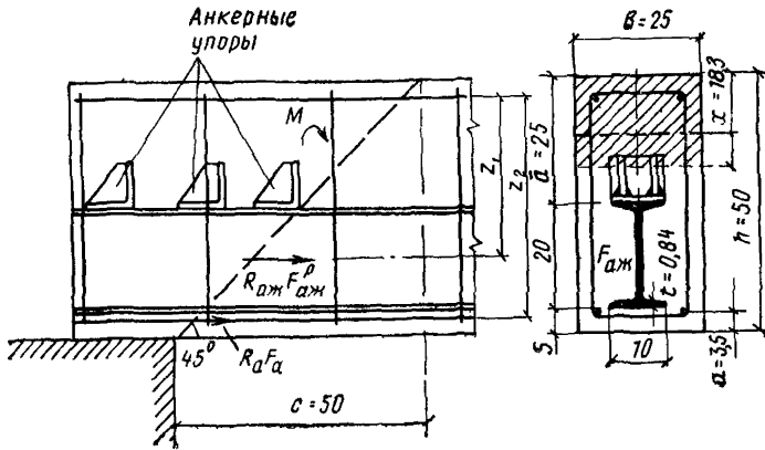
Рис. 10. К примеру расчета 7
