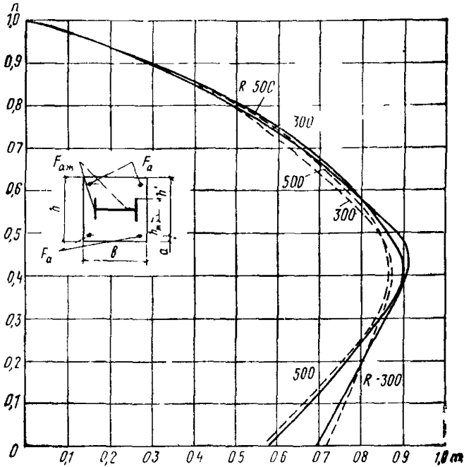
Рис. 17. График несущей способности прямоугольного сечения с жесткой арматурой в виде двутавра, стенка которого расположена перпендикулярно плоскости действия изгибающего момента.
