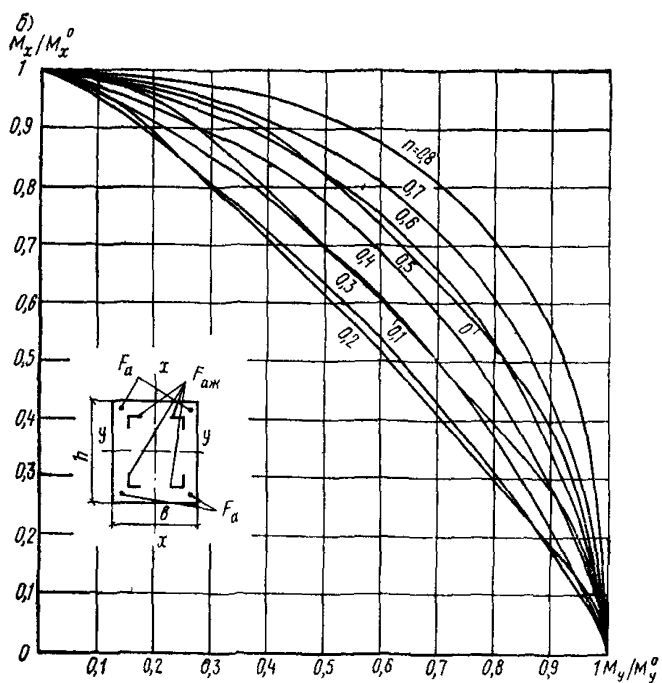
Рис. 16. График несущей способности прямоугольного сечения при косом внецентренном сжатии с жесткой арматурой а — в виде двутавра; б — в виде уголков
