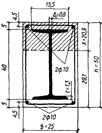
Рис. 20. К примерам расчета 11 и 12
