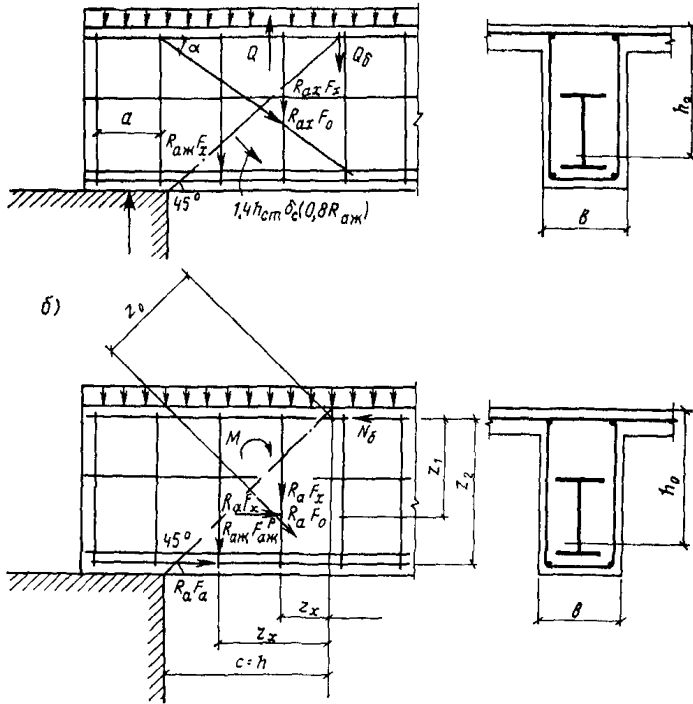
Рис. 9. Схемы усилий при расчете наклонного сечения по прочности а — по поперечной силе; б — по изгибающему моменту
