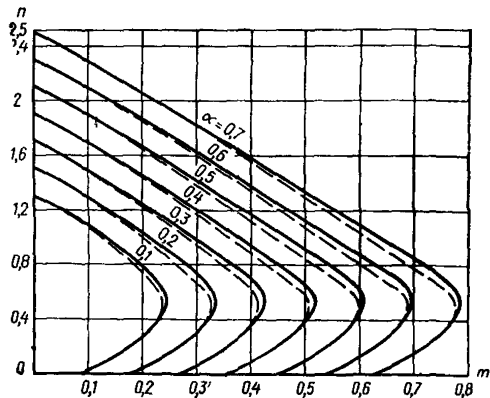
Рис. 12. График несущей способности прямоугольного сечения с жесткой и гибкой арматурой, сосредоточенной у растянутой и сжатой граней
