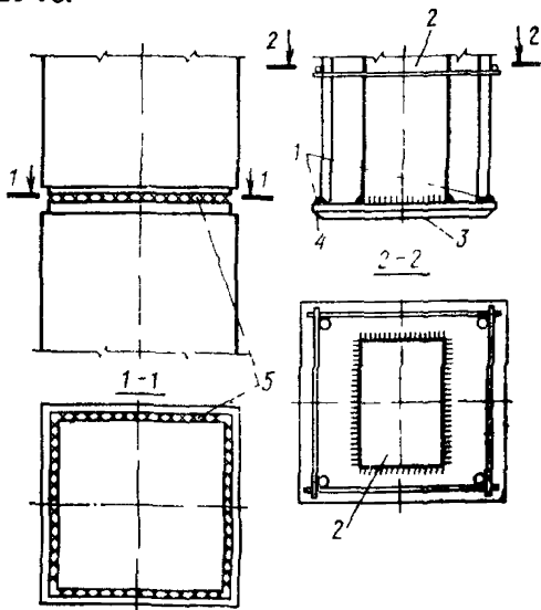
Рис. 21. Стык железобетонных колонн с жесткой арматурой типа сердечник
