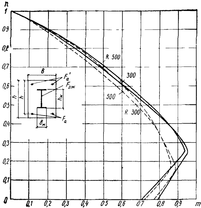
Рис. 14. График несущей способности прямоугольного сечения с жесткой арматурой в виде симметричного профиля, стенка которого расположена параллельно плоскости действия изгибающего момента (сплошные линии — сталь класса С 38/29; пунктирные — сталь класса С 48/33)
