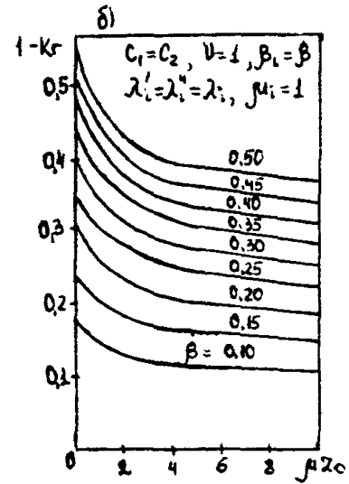
Рис. 14. Двухфазная система с равными производностями фаз
