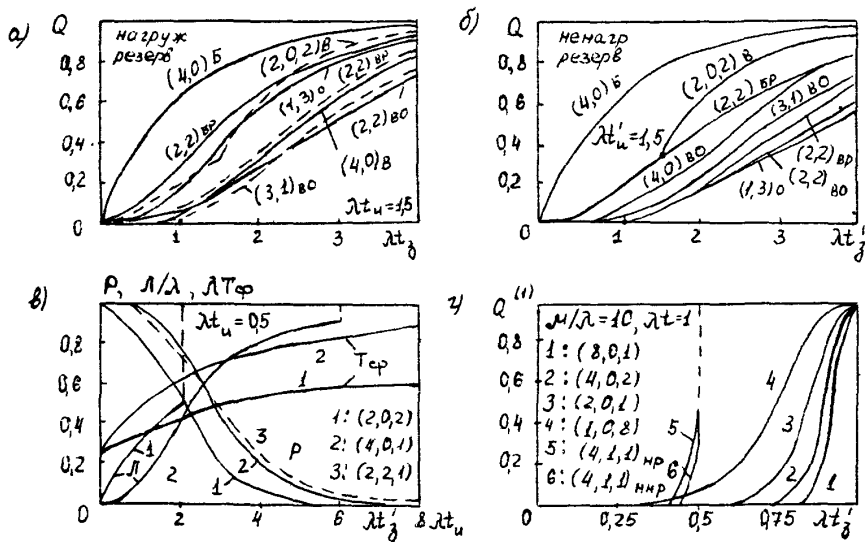
Рис. 13. Многоканальные системы с различными способами группобразования
