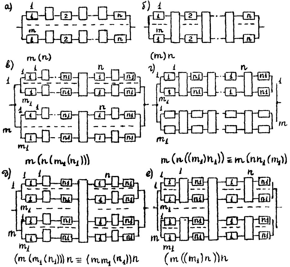
Рис.2. Варианты структур многоканальных систем.
