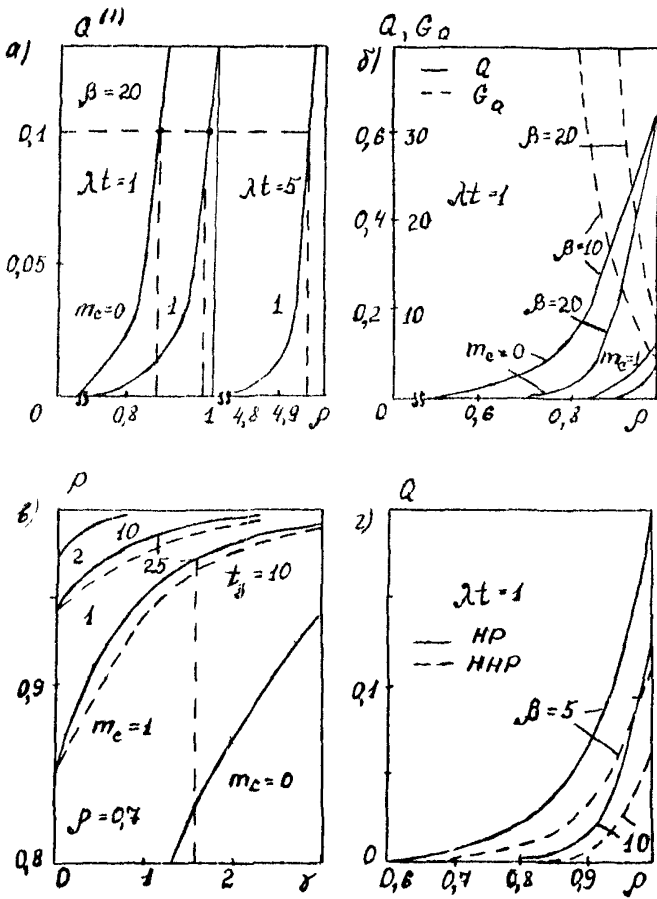
Рис. 8. Характеристики надёжности системы со структурным и временным резервированием ( — P точное, - - - P_{HP} по формуле ( 39 ) ).
