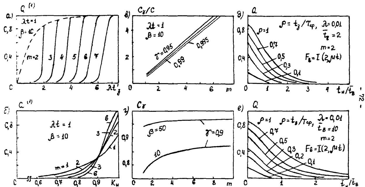
Рис. 9. Характеристики надёжности многоканальной системы с необесцениваемыми отказами
