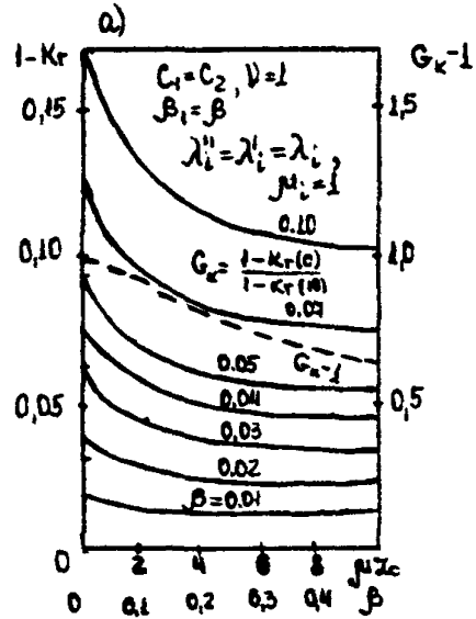
Рис. 14. Двухфазная система с равными производностями фаз
