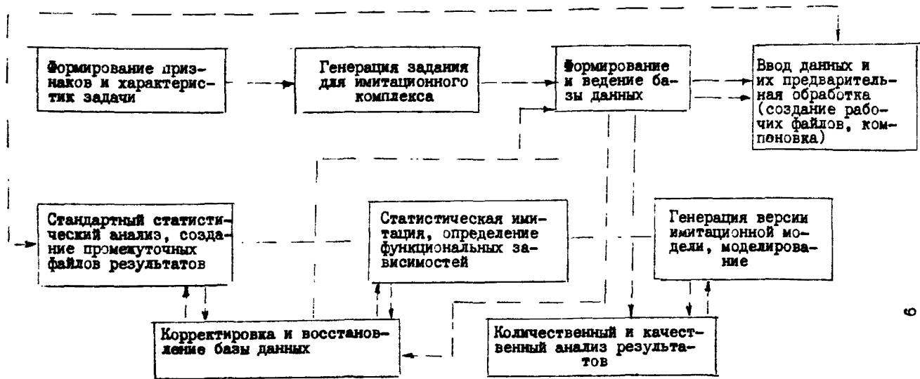
Рис. 1.3. Технологическая схема статистического анализа и моделирования объектов стандартизации.
