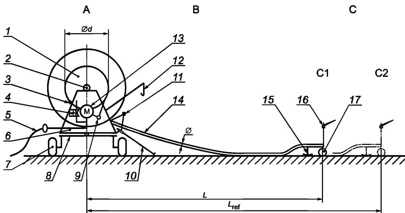
А — конструкция машины; В — раздаточная труба; С — тележка; С1 — текущее положение тележки; С2 — самое дальнее положение тележки; d — диаметр барабана; \varnothing — наружный диаметр раздаточной трубы; L_{ref} — номинальная длина раздаточной трубы; L — текущая длина движущейся части раздаточной трубы, лежащей и тянущейся по полю; 1 — барабан; 2 — вал барабана; 3 — тормоз барабана; 4 — устройство управления движением системы распределения воды; 5 — шланг для подсоединения машины к источнику воды; 6 — опора барабана (жесткая или поворотная); 7 — колесо; 8 — шасси; 9 — вал внешнего привода; 10 — стабилизирующие опоры; 11 — направляющий механизм раздаточной трубы; 12 — устройство подъема тележки; 13 — гидропривод (турбинный или поршневой) и механизм привода; 14 — раздаточная труба (обычно полиэтиленовая); 15 — полоз тележки; 16 — система распределения воды: дождевальная аппаратура, включая дождевальный аппарат пушечного типа с секторным регулированием, штанга или другое устройство; 17 — колесо тележки
