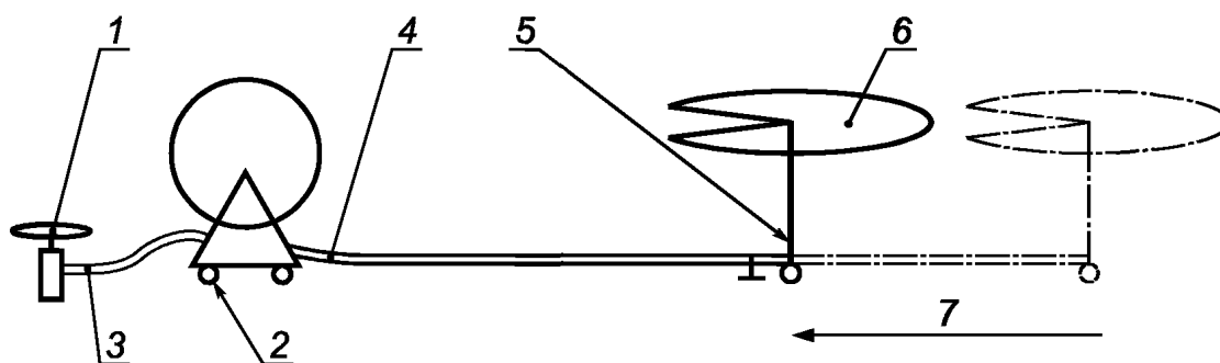
1 — источник воды; 2 — стационарный барабан; 3 — труба/шланг от источника воды; 4 — раздаточная труба (тянущего типа); 5 — тележка; 6 — устройство или система распределения воды: дождевальный аппарат, в том числе пушечного типа, штанга (на тележке); 7 — направление движения
