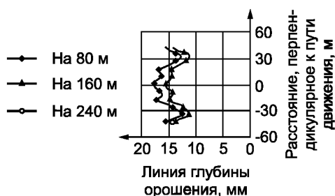
б) Глубина орошения зон перекрытия на выбранных поперечных линиях
