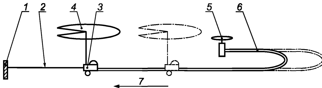
1 — якорь буксирного каната; 2 — буксирный канат; 3 — тележка; 4 — устройство или система распределения воды: дождевальный аппарат, в том числе пушечного типа, штанга (на тележке); 5 — источник воды; 6 — раздаточный шланг; 7 — направление движения
