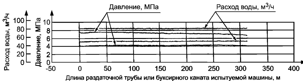
е) Отклонения давления и расхода воды
