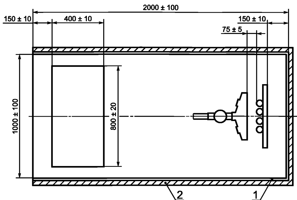
Рисунок 1 — Испытательная камера
