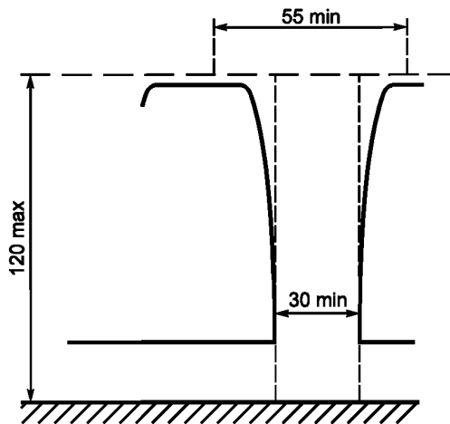
Рисунок 20 — Определение свободного доступа к двери (см. 5.7.1.10.2)
