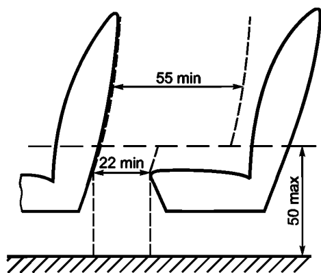
Рисунок 19 — Определение свободного доступа к двери (см. 5.7.1.10.1)
