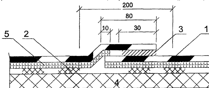
Рис. 2.9. Стык смежных полотенц термопластичной пленки
