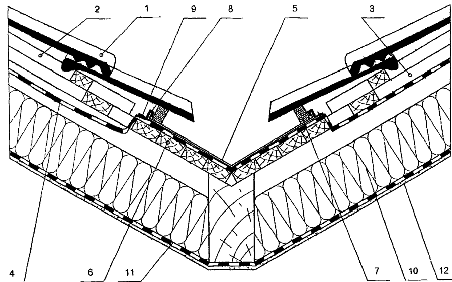
Рис 1.27. Ендовы черепичной кровли чердака (а) и крыши с диффузионно-гидроизоляционной пленкой (б)
