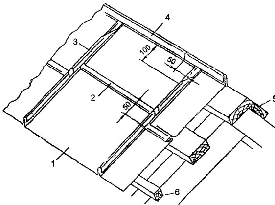
Рис. 2.49. Рядовое покрытие ската листовой сталью (медью). 1 – картина в рядовой полосе, 2 – одинарный лежащий фальц, 3 – одинарный стоячий фальц, 4 – коньковый стоячий фальц, 5 – доска, 6 – брус обрешетки.
