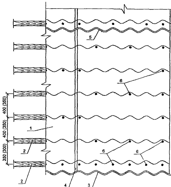
Рис. 2.45. Крепление металлочерепицы
