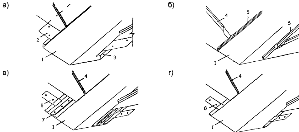
Рис. 1.64. Ендова кровли
