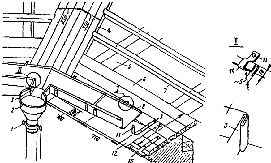
Рис. 2.51. Устройство настенного желоба
