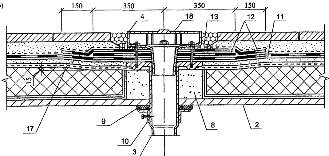
Рис. 1.1. – 1.2. Водоприемная воронка
