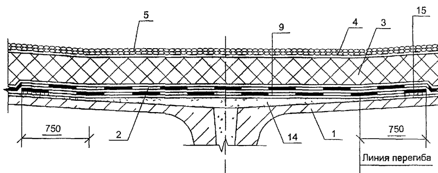
Рис. 1 14 Инверсионная кровля
