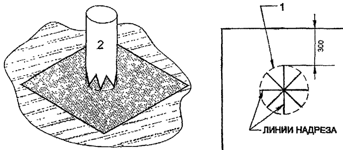
Рис. 2.18. Укладка нижнего слоя дополнительного водоизоляционного ковра 1 – линия изгиба; 2 – труба.
