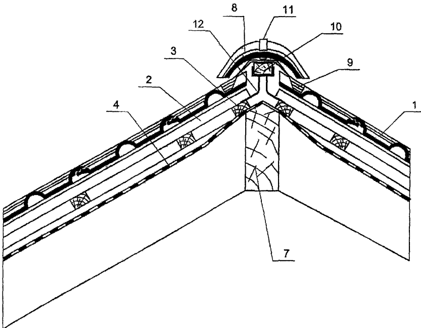
Рис. 1.28. Хребет крыши (а) и чердачной кровли (б) 1– черепица; 2 – обрешетка; 3 – контробрешетка; 4 – ветрозащитная диффузионно-гидроизоляционная пленка (см. Приложение 9); 5 – утеплитель; 6 – пароизоляция; 7 – хребтовая стропильная нога; 8 – коньковая черепица; 9 – “Фигароль” – аэроэлемент хребта (см. Приложение 7); 10 – хребтовый брусок; 11 – зажим (кляммер) коньковой черепицы (см. Приложение 8); 12 – крепление хребтового бруска; 13 – внутренняя обшивка
