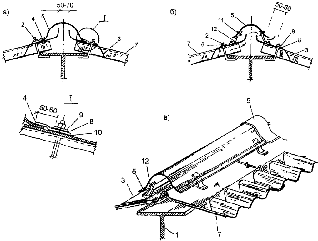
Рис 1 49. Коньковые узлы по металлическим прогонам а – глухой конек; б и в – конек с вентиляционными щелями, 1 – прогон; 2 – крюк; 3 – малая переходная деталь; 4 – прижимная скоба; 5 – коньковая деталь; 6 – гайка; 7 – лист; 8 – резиновая прокладка; 9 – стальная шайба; 10 – резиновая прокладка; 11 – заклепка; 12 – стальная стойка.
