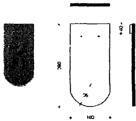
Рис. 1.17. План черепицы, поперечный и продольный разрезы.
