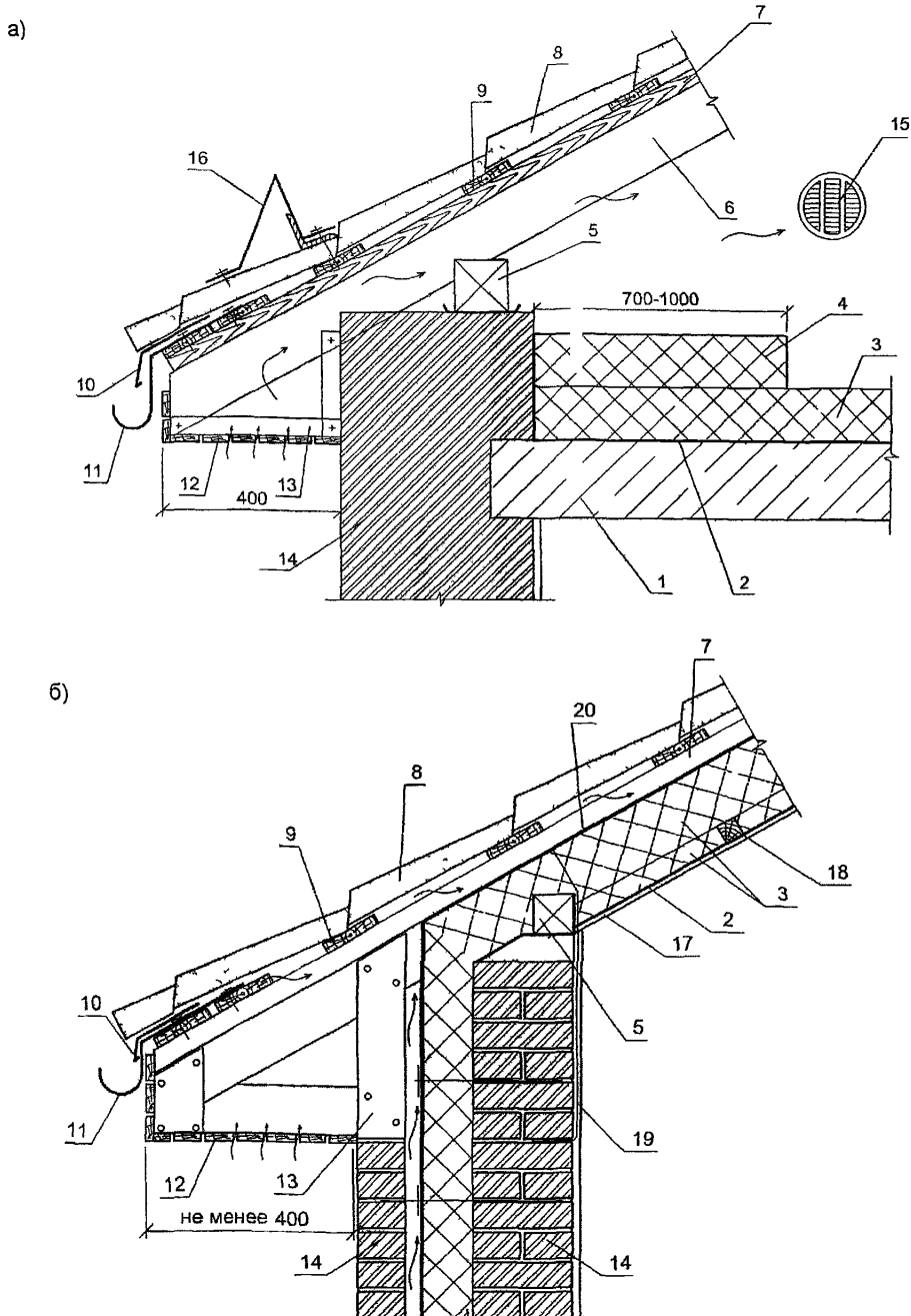
Рис 1 39 Карнизный узел кровли холодного чердака (а) и крыши мансарды (б) 1 – несущая плита, 2 – пароизоляция, 3 – теплоизоляция, 4 – дополнительная теплоизоляция по периметру здания, 5 – мауэрлат, 6 – стропило, 7 – контробрешетка, 8 – металлочерепица, 9 – обрешетка, 10 – карнизная планка (капельник) (см Приложение 11), 11 – скоба желоба, 12 – подшивка карниза, 13 – каркас карнизного свеса, 14 – стена, 15 – щипцовое окно, 16 – снеговой барьер (см Приложение 11), 17 – гипсокартон, 18 – брусок, 19 – анкер стропила и мауэрлата, 20 – ветрозащитная диффузионно-гидроизоляционная пленка (см Приложение 9)
