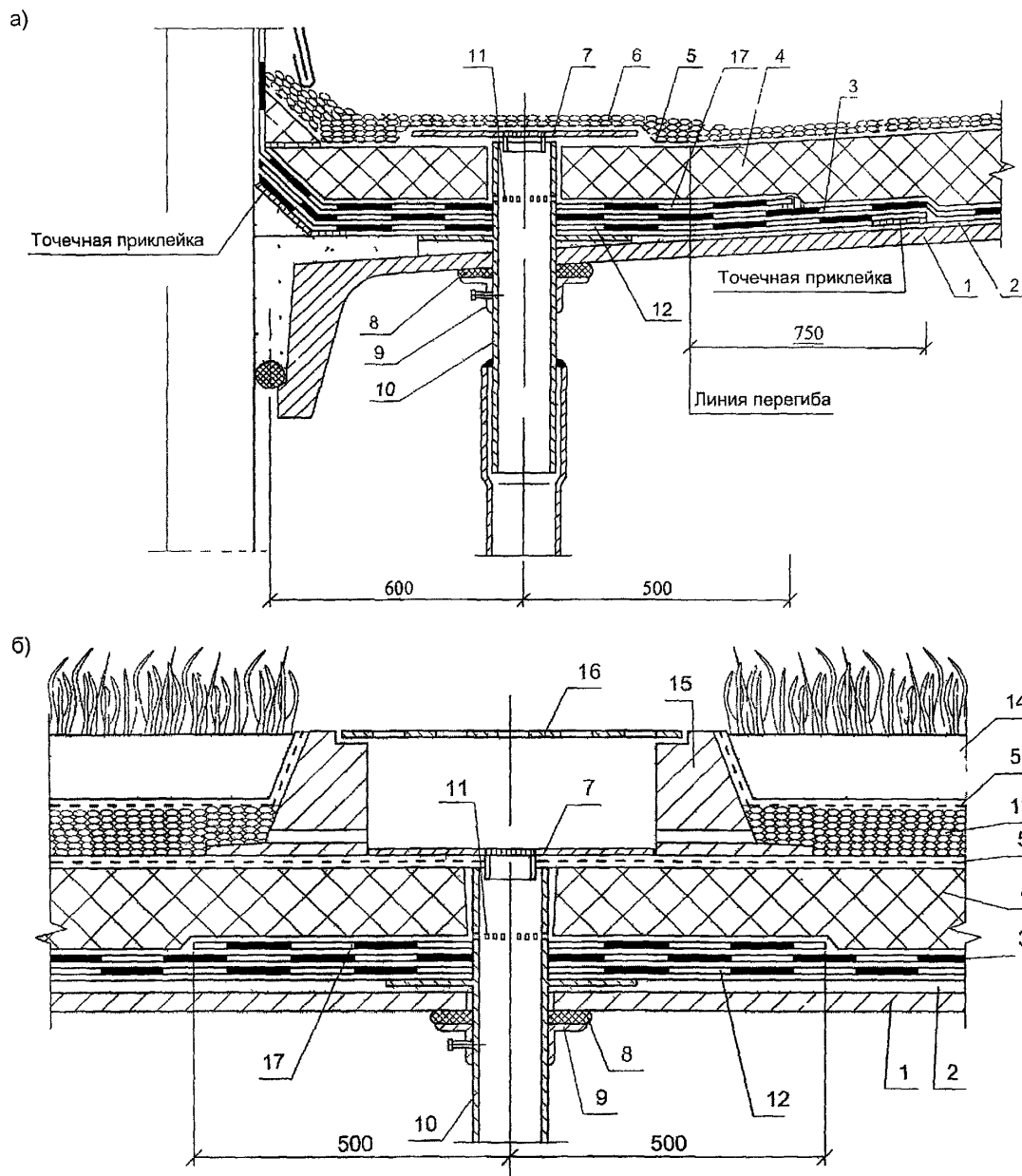
Рис 1 12 Воронка внутреннего водостока инверсионной кровли с гравийным пригрузом (а) и травяным растительным покровом (б)
