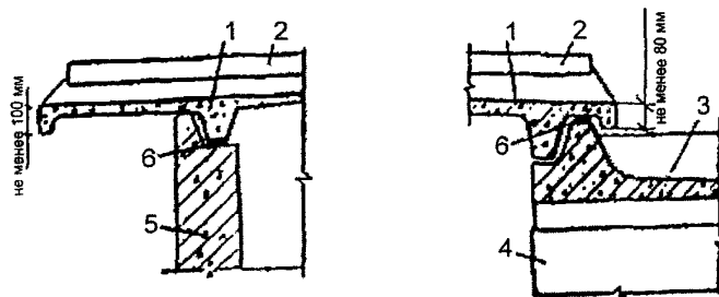
Рис. 1.67. Конструкции свесов
