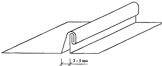
Рис. 1.60 Компенсационный стык
