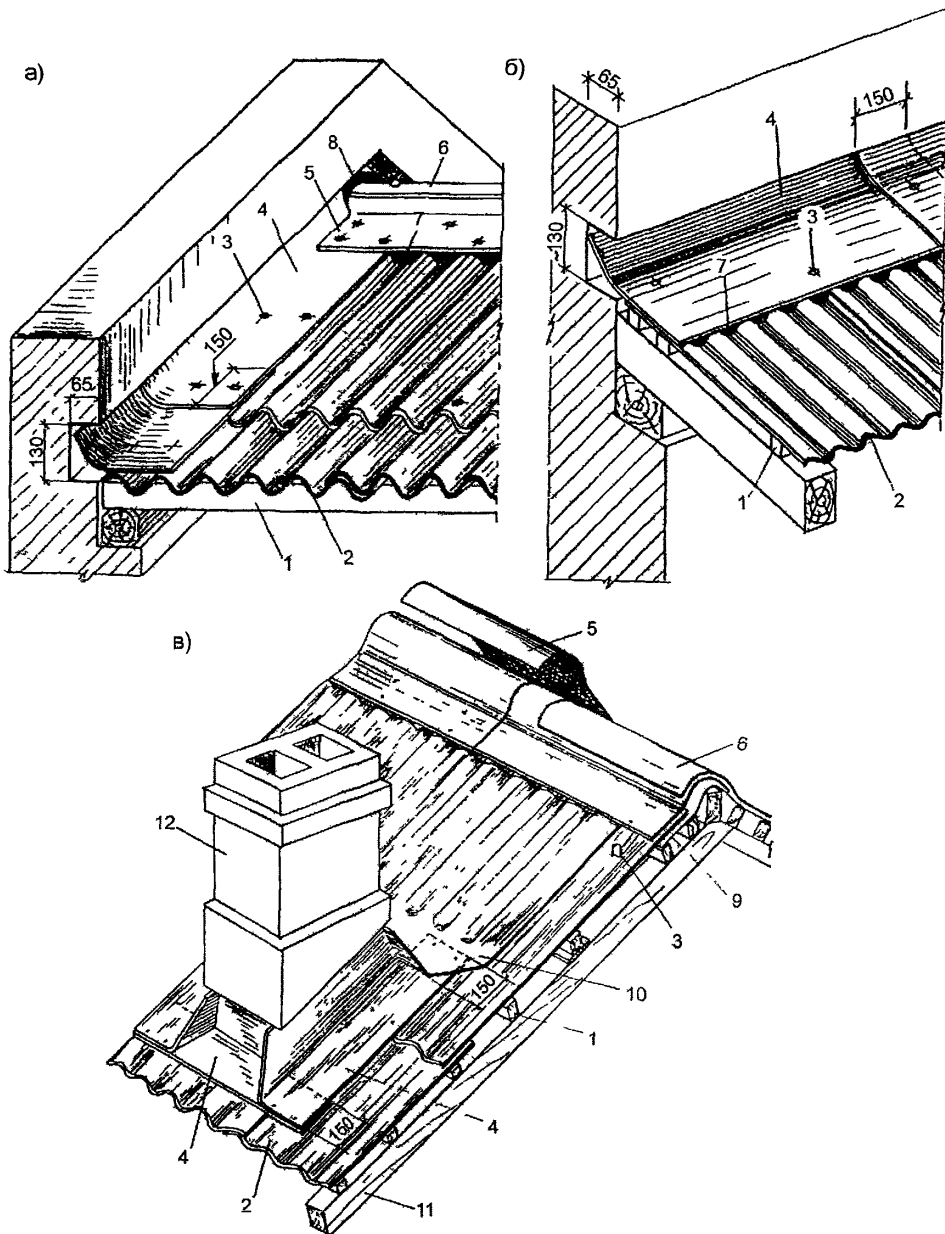
Рис 1 46 Примыкание кровли из асбестоцементных волнистых листов к поперечной (а) и продольной (б) стенам и к дымовой трубе (в) 1 – обрешетка, 2 – асбестоцементный лист, 3 – скоба, 4 – уголковая деталь, 5 – коньковая деталь, 6 – конек, 7 – уплотнитель, 8 – заделка раствором, 9 – прокладка из рулонного водоизоляционного материала, 10 – затрубный уголок, 11 – стропильная нога, 12 – оголовок дымовой трубы
