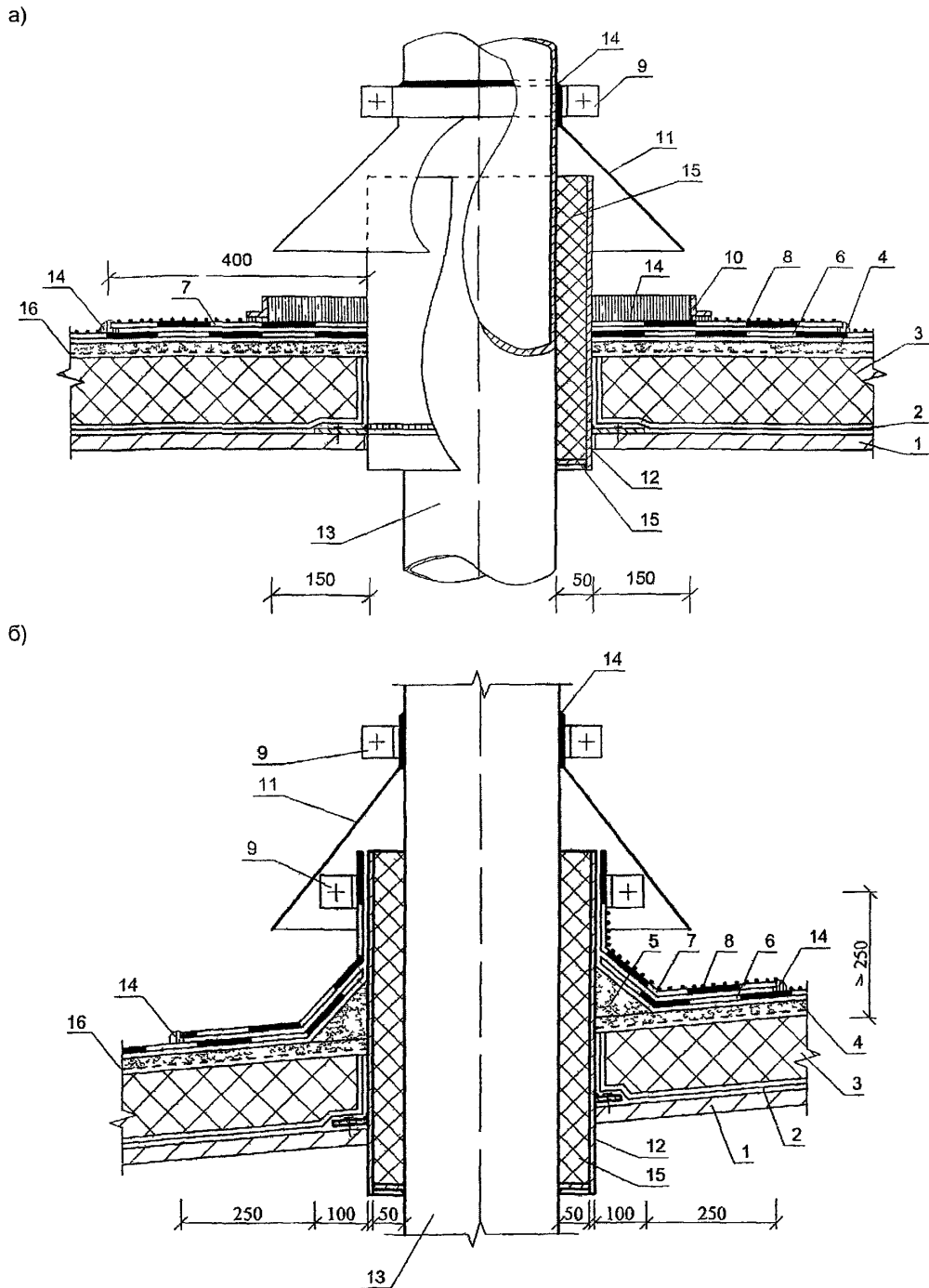
Рис 17 Пропуск трубы через покрытие с традиционной кровлей а) с герметизацией мастикой, б) с устройством бортиков из раствора, 1 – сборная железобетонная панель, 2 – пароизоляция, 3 – теплоизоляция, 4 и 5 – выравнивающая стяжка и бортик из цементно-песчаного раствора, 6 – основной водоизоляционный ковер, 7 – дополнительные слои водоизоляционного ковра, 8 – защитный слой (крупнозернистая посыпка), 9 – хомут, 10 – рамка из стального уголка, 11 – зонтик из оцинкованной стали, 12 – патрубок с фланцем, 13 – труба, 14 – герметизирующая мастика, 15 – стекловата, 16 – разделительный слой
