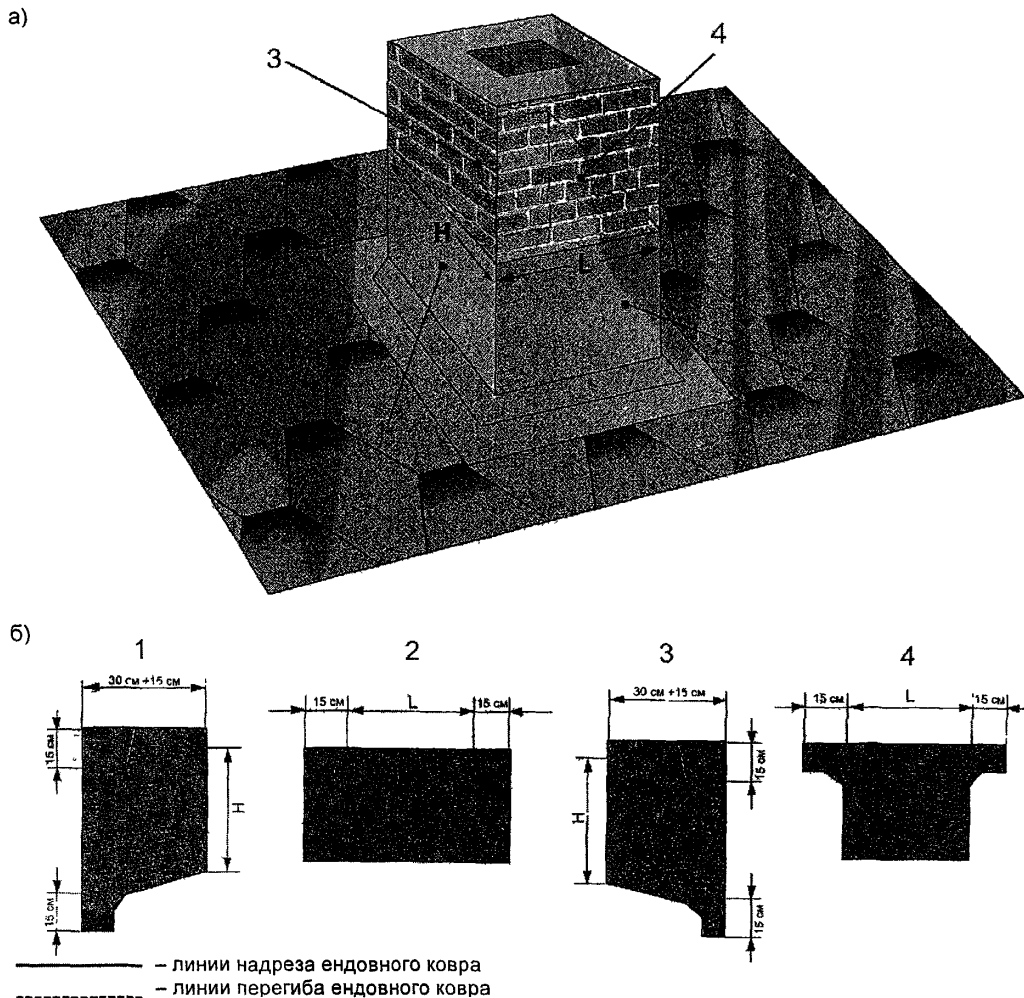
Рис. 2.43. Примыкание кровли из гибкой черепицы к дымовой трубе (а) и раскрой рулонного материала по сторонам трубы (б)
