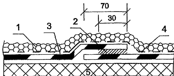
Рис. 2.10. Стык смежных полотенц термопластичной пленки
