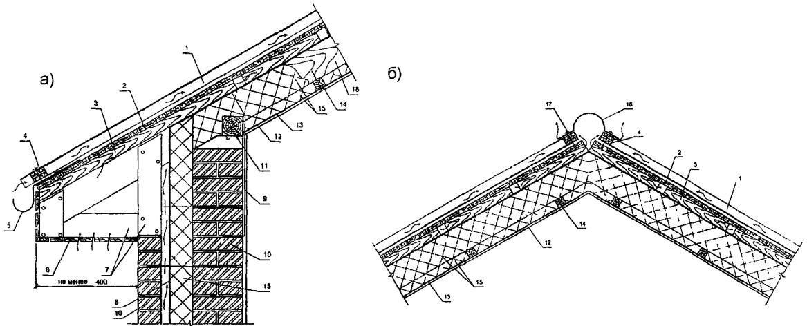
Рис. 1 50 Карнизный (а) и коньковый (б) узлы кровли 1 – битумный волнистый лист; 2 – обрешетка (сплошной настил); 3 – контробрешетка; 4 – уплотнитель с вентиляционными отверстиями (см. Приложение 12); 5 – скоба для лотка; 6 – подшивка карниза; 7 – каркас карнизного свеса; 8 – ветрозащитная диффузионно- гидроизоляционная пленка (см. Приложение 9); 9 – анкер крепления стропила и мауэрлата; 10 – стена; 11 – мауэрлат; 12 – гипсокартон; 13 – пароизоляция; 14 – брусок; 15 – теплоизоляция; 16 – коньковый элемент; 17 – гвоздь с закрывающейся шляпкой (см Приложение 12)
