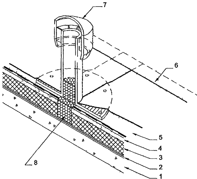
Рис 2 28 Патрубок 1 – несущая плита, 2 – пароизоляция, 3 – теплоизоляция, 4 – выравнивающая стяжка, 5 – частично приклеенный рулонный материал, 6 – верхний слой кровельного ковра, 7 – патрубок, 8 – заполнение керамзитовым гравием
