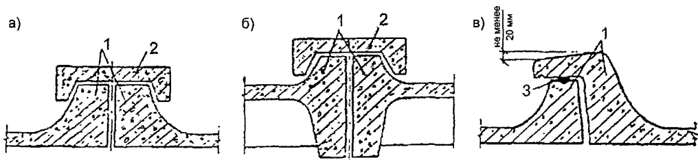
Рис. 1.66. Конструкции стыков кровельных панелей а, б – стык с перекрытием П-образным нащельником; в – стык внахлестку; 1 – кровельная панель; 2 – П-образный нащельник; 3 – герметик (прокладка «виларем»).
