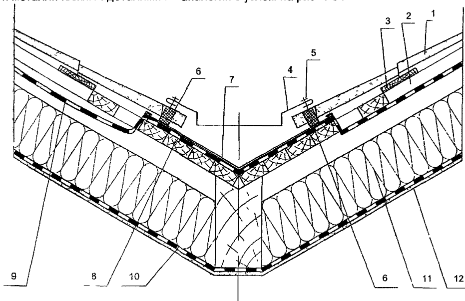
Рис. 1 42. Ендова кровли
