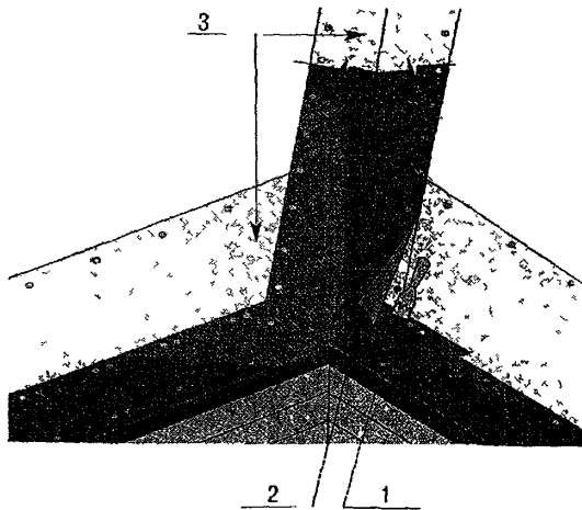
Рис 2 37 Ендова кровли 1 – промазка битумной мастикой, 2 – ендовый ковер, 3 – подкладоч- ные слои
