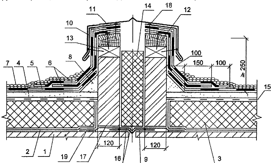
Рис. 1.4. Деформационный шов
