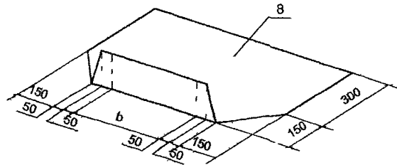
Задний уголок (b - ширина трубы)
