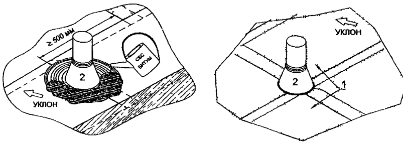
Рис 2 25 Обклейка трубы вторым слоем основного водоизоляционного ковра 1 – полотноца второго слоя основного ковра, 2 – труба
