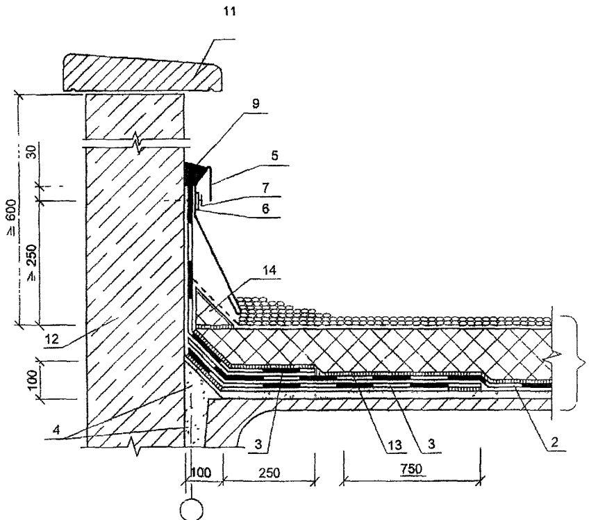
Рис 1 13 Примыкание инверсионной кровли к парапету а) парапет высотой до 450 мм; б) парапет высотой более 450 мм, 1 – покрытие по типу К-4 (см. табл 1), 2 – основной водоизоляционный ковер, 3 – дополнительные слои водоизоляционного ковра; 4 – бортик и заполнение из бетона, 5 – защитный фартук из оцинкованной стали толщиной 0,8 мм, 6 – стальная полоса 40×4 мм, 7 – дюбельный гвоздь, 8 – костыль, 9 – мастика герметизирующая, 10 – ограждение; 11 – плита парапетная; 12 – стена, 13 – сплошная приклейка плит утеплителя в зоне парапета (на ширину 1,5 м), 14 – доборный утеплитель
