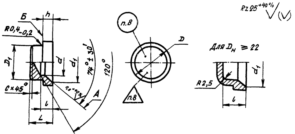
Размеры, мм
