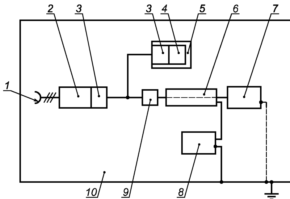
1 — сеть электропитания переменного тока 220 В, 50 Гц; 2 — блок питания; 3 — фильтр; 4 — передатчик / приемник; 5 — блок связи; 6 — емкостные клещи связи; 7 — испытуемый блок; 8 — испытательный генератор НИП; 9 — аттенюатор; 10 — пластина заземления
