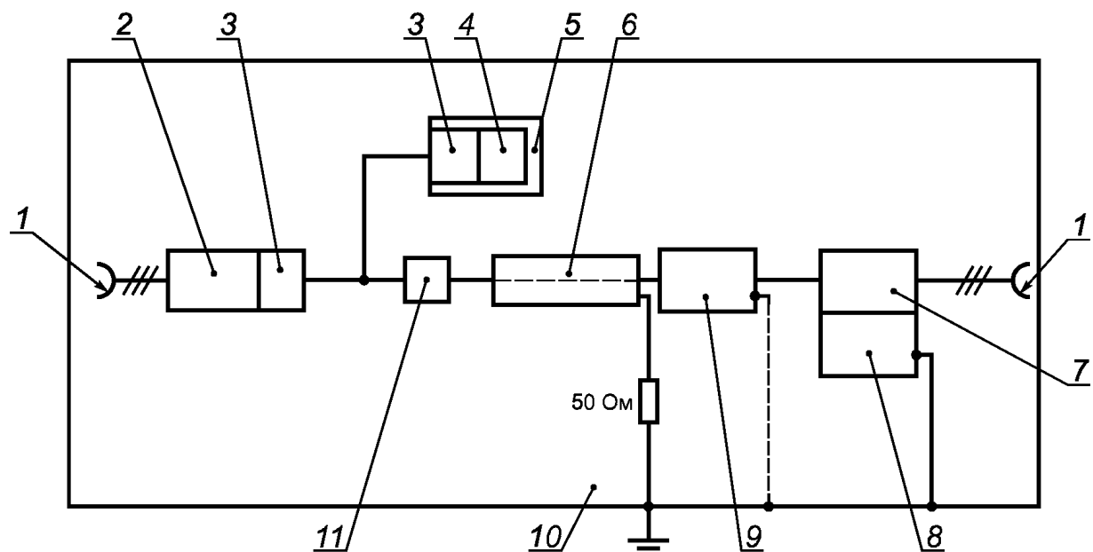
1 — сеть электропитания переменного тока 220 В, 50 Гц; 2 — блок питания; 3 — фильтр; 4 — передатчик / приемник; 5 — блок связи; 6 — емкостные клещи связи; 7 — устройство связи / развязки; 8 — испытательный генератор НИП; 9 — испытуемый блок; 10 — пластина заземления; 11 — аттенюатор
