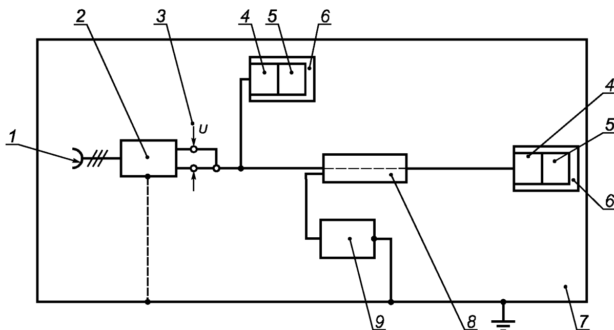
Рисунок 3 — Схема испытаний блока питания при подаче НИП на порт электропитания переменного тока
