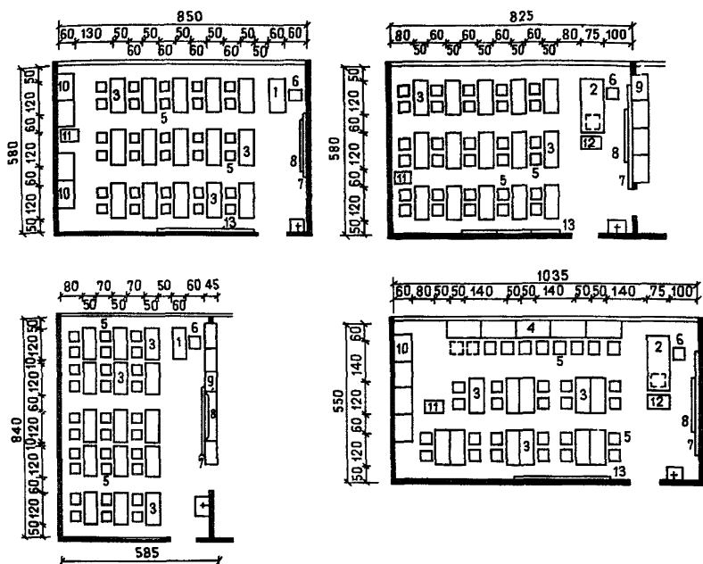
Рис. 18. Планировка кабинетов общеобразовательного цикла
