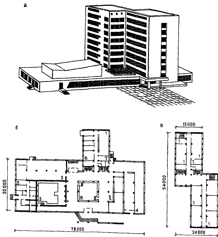
Рис. 65. Учебный комбинат на 1950 мест (ЦНИИЭП учебных зданий, арх. Г. Лапир, Н. Смирнова, А. Гарнец) а - общий вид; б - план первого этажа; в - план типового этажа; 1 - учебные помещения; 2 - вестибюль; 3 - конференц-зал; 4 - лекционная аудитория; 5 - столовая; 6 - административные помещения; 7 - препараторская; 8 - внутренний дворик
