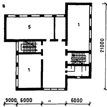
Рис. 61. Учебный пункт на 200 мест (ЦНИИЭП учебных зданий, арх. Г. Лапир, Л. Кривуценок)
