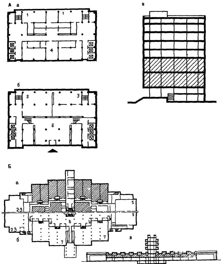
Рис. 12. Функциональная структура многоэтажных зданий А - проект ПТУ в М скве (ЦНИИЭП учебных зданий); а - план типового этажа; б - план первого этажа; Б - ремесленное училище в г. Амстерфотте (Голландия);
