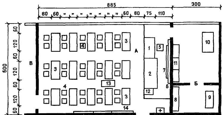
Рис. 23. Планировка кабинета начальной военной подготовки А - учебный кабинет ; Б - комната хранения оружия ; В - препарат- торская ; 1 - стол преподавателя ; 2 - стол демонстрационный ; 3 - стол ученический ; 4 - стул учащегося ; 5 - стул преподавате- ля ; 6 - доска меловая ; 7 - экран ; 8 - шкаф ; 9 - стеллаж ; 10 - стол для чистки оружия ; 11 - шкаф для учебных пособий и материалов ; 12 - тумба для графопроектора ; 13 - тумба для про- екционных аппаратов ; 14 - щит экспозиционный
