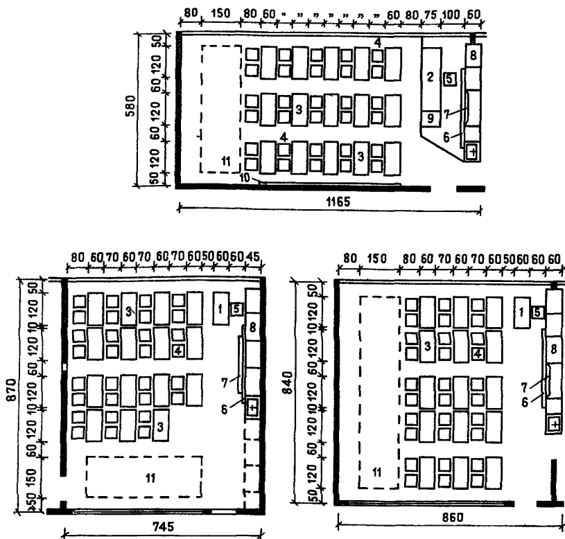
Рис. 21. Планировка кабинетов профессионально-технического, общетехнического, специального циклов
