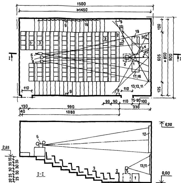
Рис. 35. Лекционная аудитория на 120 мест размерами 9x15 м 1 - стол преподавателя; 2 - стол-пюпитр; 3 - кресло с пюпитром; 4 - кресло преподавателя; 5 - графопроектор; 6 - кинопроектор; 7 - диапроектор; 8 - автоматический проектор; 9 - звуковая колонка; 10 - экран для проекции на просвет; 11 - экран для графопроектора; 12 - экран стационарный; 13 - доска меловая; 14 - доска меловая раздвижная; 15 - зеркало для проекции; 16 - зашторивание; 17 - магнитофон; 18 - проигрыватель; 19 - кафедра-трибуна
