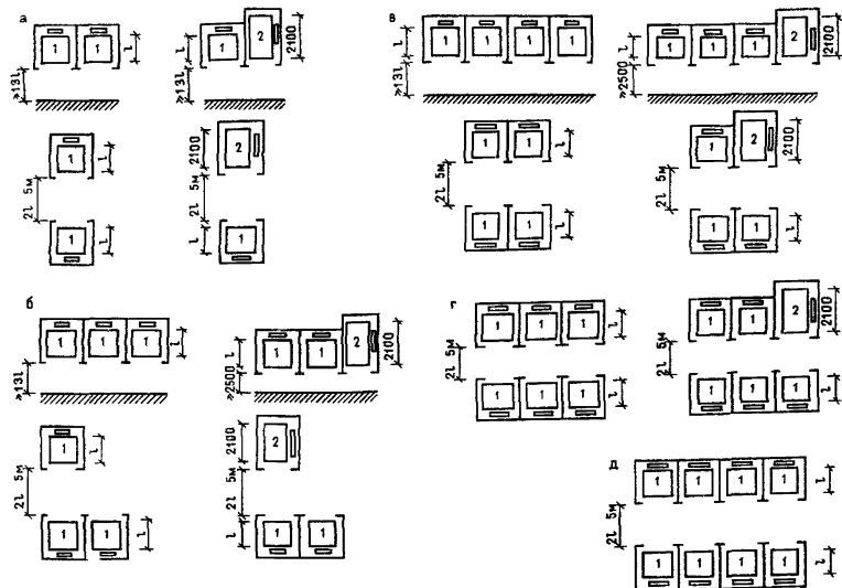
Рис. приложения 1. Сочетание и расположение группы лифтов с типовой системой группового управления
