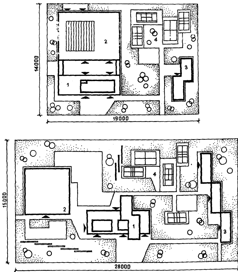
Рис. 58. Примерные схемы генпланов учебных комбинатов а - на 200 ученических мест ; б - на 900 ученических мест ; в - на 1300 ученических мест ; г - на 1950 ученических мест ; 1 - зда- ние учебного комбината ; 2 - учебные мастерские ; 3 - общежитие ; спортплощадки
