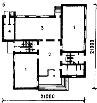
Рис. 61. Учебный пункт на 200 мест (ЦНИИЭП учебных зданий, арх. Г. Лапир, Л. Кривуценок)
