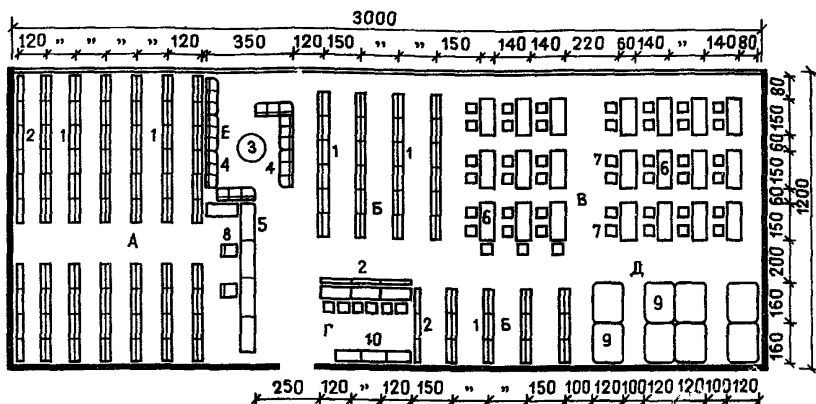
Рис. 45. Планировка и оборудование помещений библиотеки ПТУ на 720 учащихся
