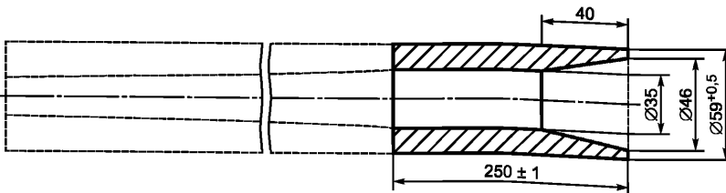
Рисунок Е.8 — Полиуретановая трубка из материала В
