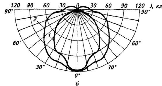
а – ЛПО 56, б – ФПО04-2x18, 1 – в продольной плоскости, 2 – в поперечной плоскости
