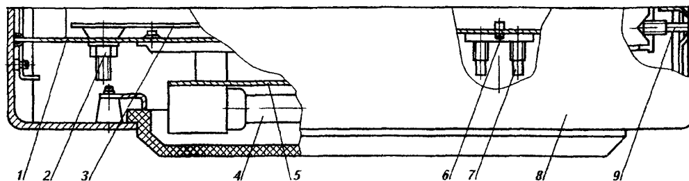
1 – основание, 2 – гайка, 3 – пластина, 4 – лампа, 5 – отрагатель, 6 – винт заземления; 7 – клеммная колодка; 8 – кожух, 9 – винт
