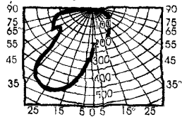
Кривые распределения силы света
