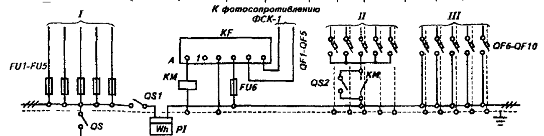
Рис 3 Электрическая принципиальная схема главного щита ввода и учета ГЩВУ-I I - квартирные магистрали, II - центральное включение фотовыключателей хозяйственного освещения, III - местное включение хозяйственного освещения, FU-FU6 - предохранители, QF1-QF10 - автоматические выключатели, KF - фотореле, QS1, QS2 - выключатели
