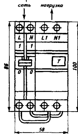
Рис. 2 Общий вид, габаритные и установочные размеры устройства защитного отключения УЗО20-ВАД1 Масса - не более 0,3 кг
