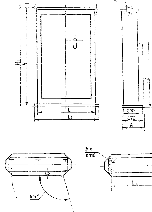
Рис.2 Напольное исполнение
