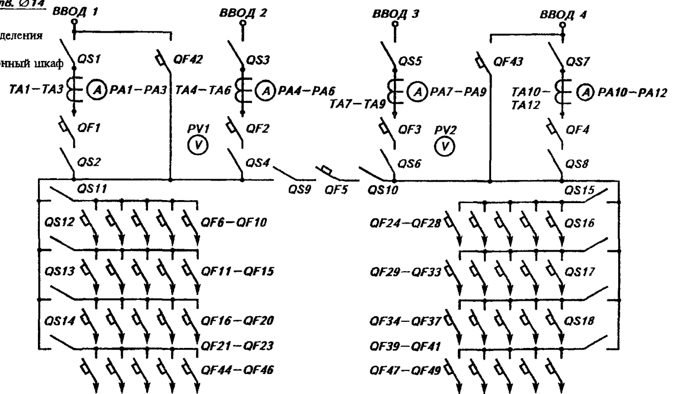
Рис 4 Электрическая принципиальная схема силовой части щитов распределения электроэнергии с АВР типа ЩР-12М РА1-РА12 - амперметры, PV1, PV2 - вольтметры, ТА1-ТА12 - трансформаторы тока, QF1-QF49 - автоматические выключатели, QS1-QS18 - разъединители
