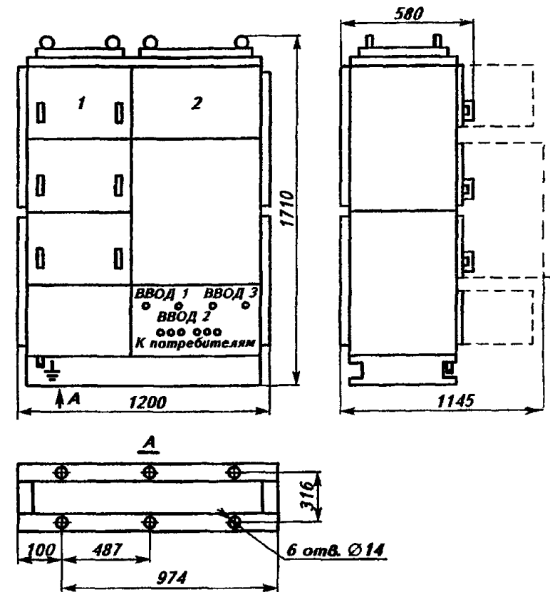
Рис. 1. Общий вид, габаритные и установочные размеры щитов распределения электроэнергии с АВР типа ЩР-12А. 1 — шкаф управления; 2 — силовой шкаф
