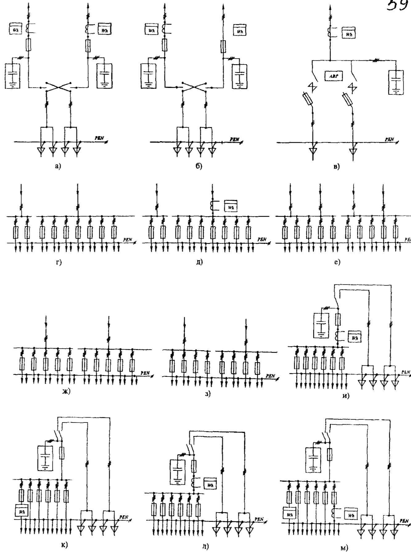
Рис 2 (1.7) Схемы вводных, распределительных, вводно-распределительных панелей ВРУ1
