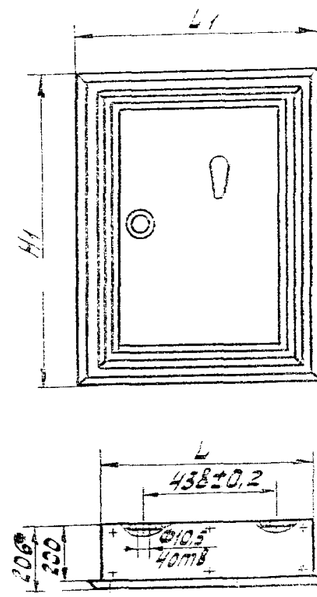
Рис.3 Утепленное исполнение
