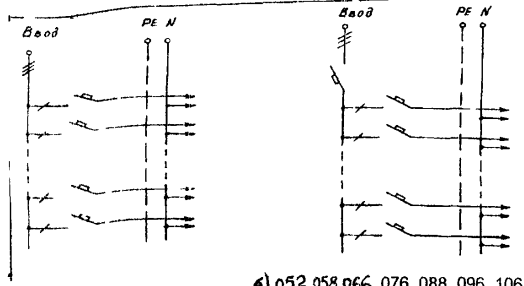
а) схемы 051 057 065, 075 б) 052, 058, 066, 076, 088 096 106
