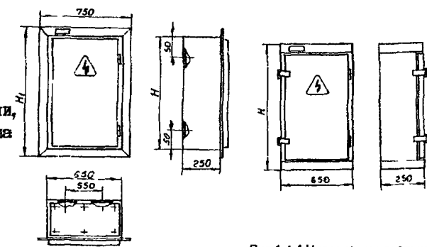
Рис 1 4 2 Утопленное исполнение IP21 Рис 1 4 4 Навесное и напольное исполнение IP54
