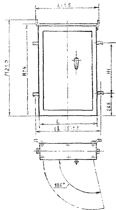
Рис.1 Навесное исполнение
