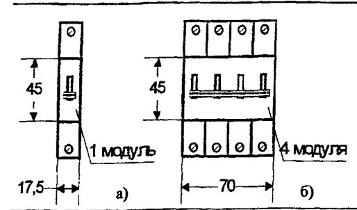
Рис.1 а) 1-модуль-однополюсный автоматический выключатель б) 4-модуля-четырёхполюсный автоматический выключатель
