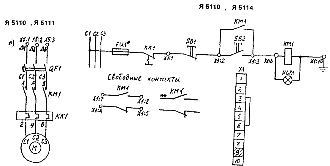
Схемы электрические принципиальные цепи силовых и управляющих ящиков типа Я 5110, Я 5111
