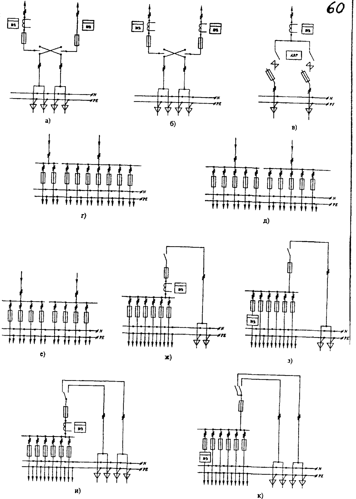
Рис. 4 Схемы вводных, распределительных, вводно-распределительных панелей ВРУЗ
