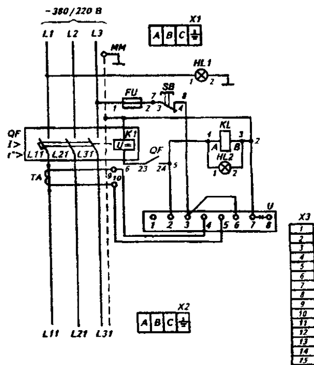
Рис 4 Электрическая принципиальная схема ящика на 25 А с клеммными колодками обозначения - по рис 4 и 5 ( см рис. 3)
