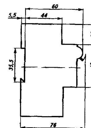
Рис. 3 Общий вид, габаритные и установочные размеры устройства защитного отключения УЗО20-ВАД2
