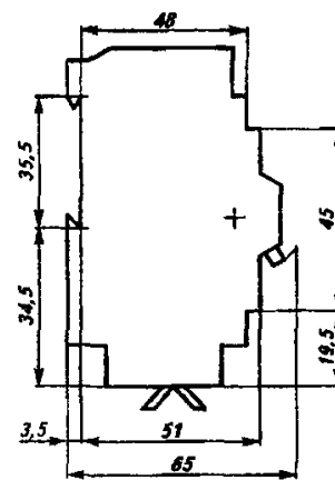
Рис. 2 Общий вид, габаритные и установочные размеры устройства защитного отключения УЗО20-ВАД1 Масса - не более 0,3 кг
