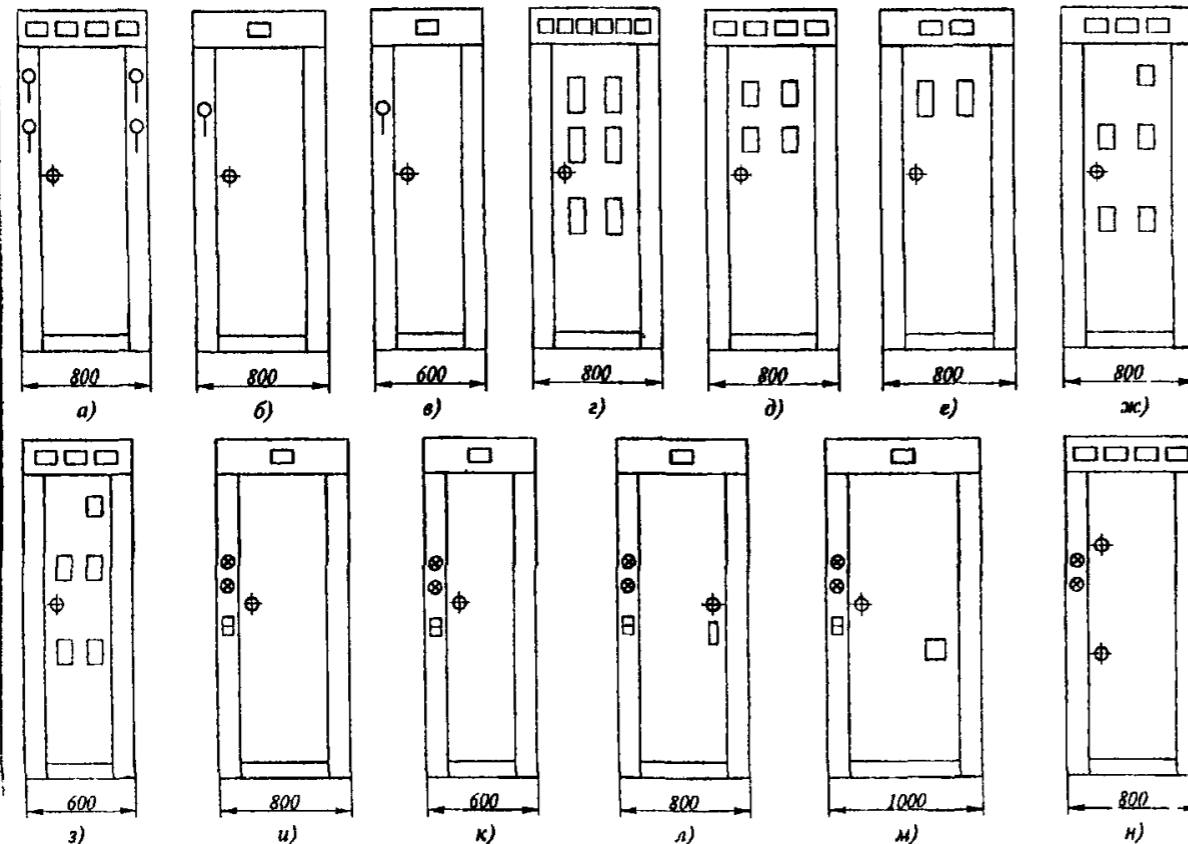
Рис 1 Фасады линейных панелей
