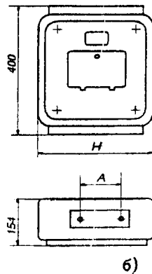
Рис. 4 Общий вид осветительных щитков: а) щитки ОП и ОПВ; б) щитки ОЩ и ОЩВ
