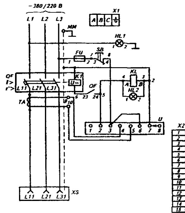
Рис 5 Электрическая принципиальная схема ящика на 63 А с одной розеткой ( см рис. 1) KL - промежуточное реле, QF - автоматический выключатель PU - предохранитель, SB - кнопка, HL1 HL2 - сигнальные лампы, TA - трансформатор тока, U - модуль защитного отключения MM - зажим заземления корпуса, X1, X2 - клеммные колодки, XS - розетка
