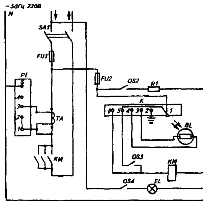
Рис 1 Электрическая принципиальная схема шкафа типа ШОУ-1 BL — фоторезистор, EL — лампа накаливания, FU1, FU2 — предохранители, K — фотореле, KM — магнитный пускатель, PI — счетчик, R1 — резистор, SA1 — рубильник, QS2-QS4 — выключатели, TA — трансформатор тока
