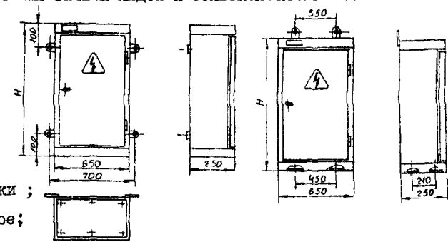
Рис 1 4 1 Навесное исполнение IP21 Рис 1 4 3 Напольное исполнение IP21
