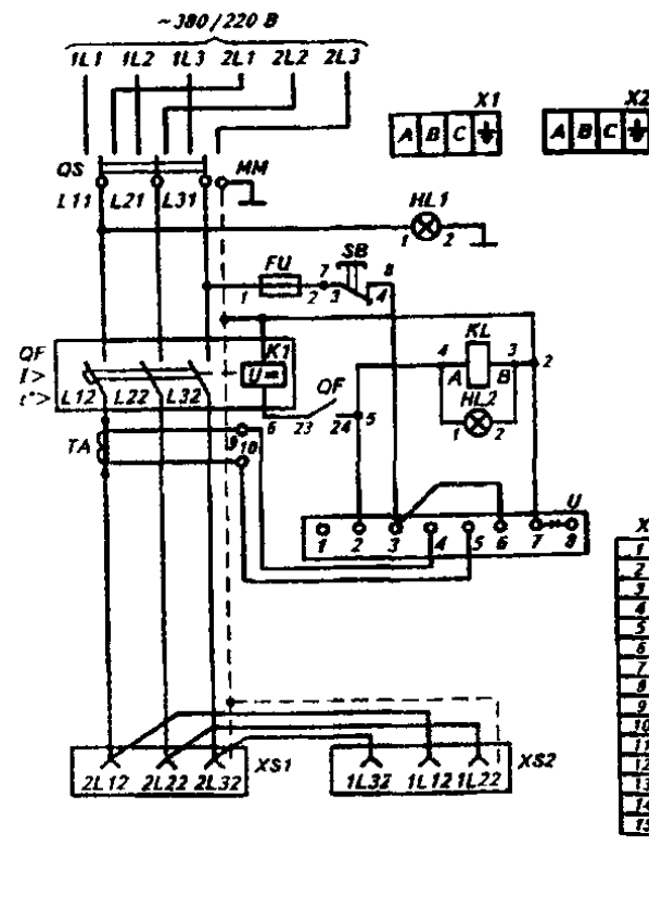
Рис 6 Электрическая принципиальная схема ящика на 63 А с двумя розетками и переключателем ( см рис 2) X1 X2 - розетки X3 - клеммная колодка, остальное - по рис 4
