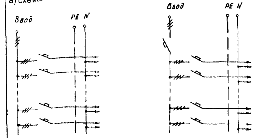
в) схемы 053 059 067 077 г) схемы 054, 060, 068, 078, 090 098, 108, 118
