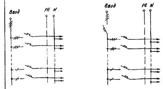
д) схемы 055, 061 063 069 071 ж) схемы 056, 062 064, 070, 072, 074, 080 082 084 073 079 081 083, 085 з) схемы 056, 062 064, 070, 072, 074, 080 082 084 086 092, 094 100, 102, 104 110 112 114, 116
