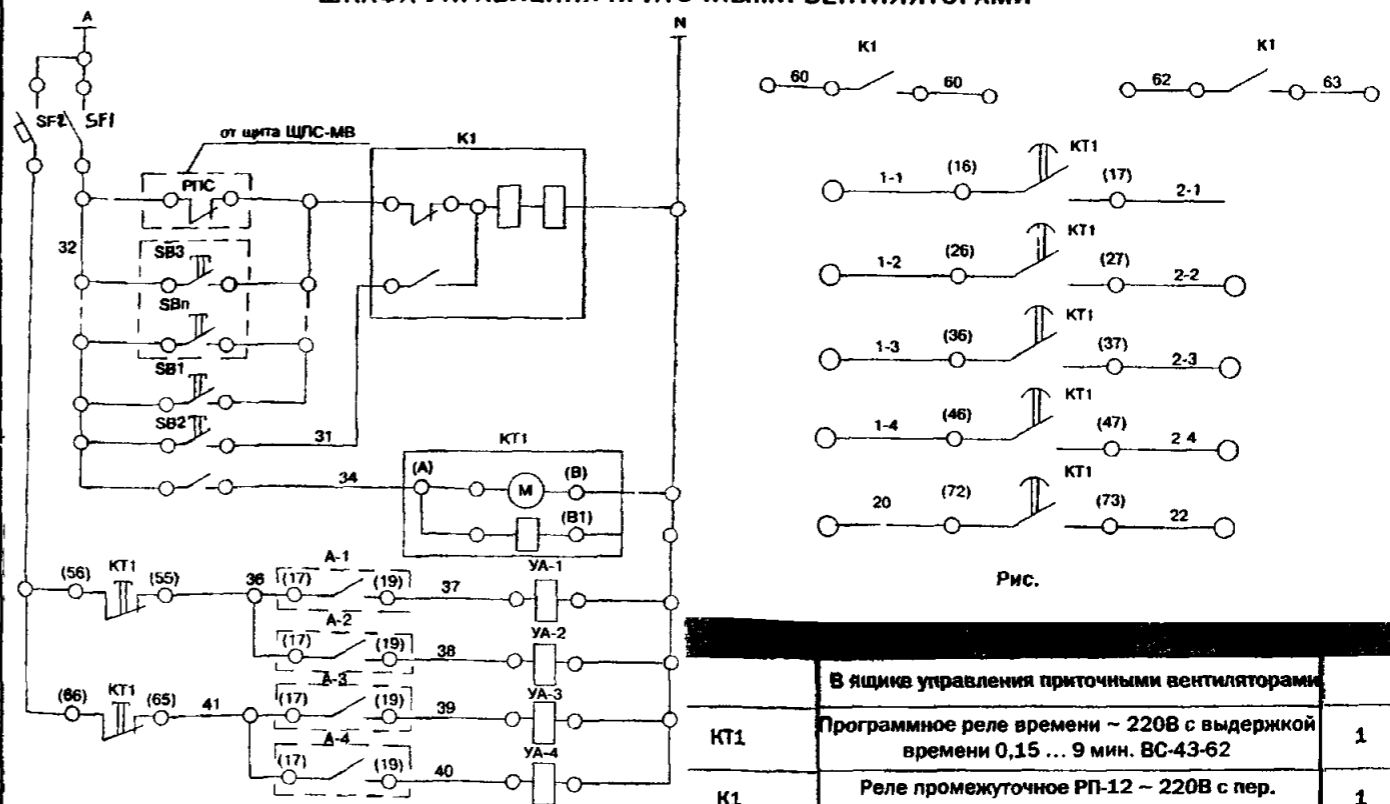
ПРИНЦИПАЛЬНАЯ ЭЛЕКТРИЧЕСКАЯ СХЕМА ШКАФА УПРАВЛЕНИЯ ПРИТОЧНЫМИ ВЕНТИЛЯТОРАМИ
