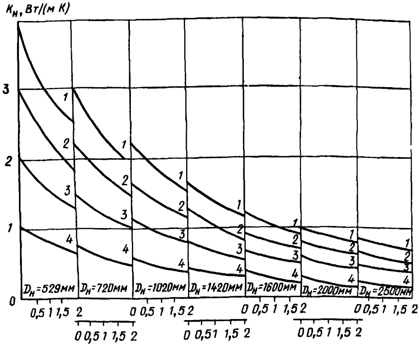
Рис. 1. Номограмма для определения коэффициента теплопередачи подземного трубопровода k_n в зависимости от глубины заложения трубопровода h_g и внешнего диаметра трубопровода D_n 1 - \lambda = 2 Вт/(м·К); 2 - \lambda = 1,5 Вт/(м·К); 3 - \lambda = 1 Вт/(м·К); 4 - \lambda = 0,5 Вт/(м·К)
