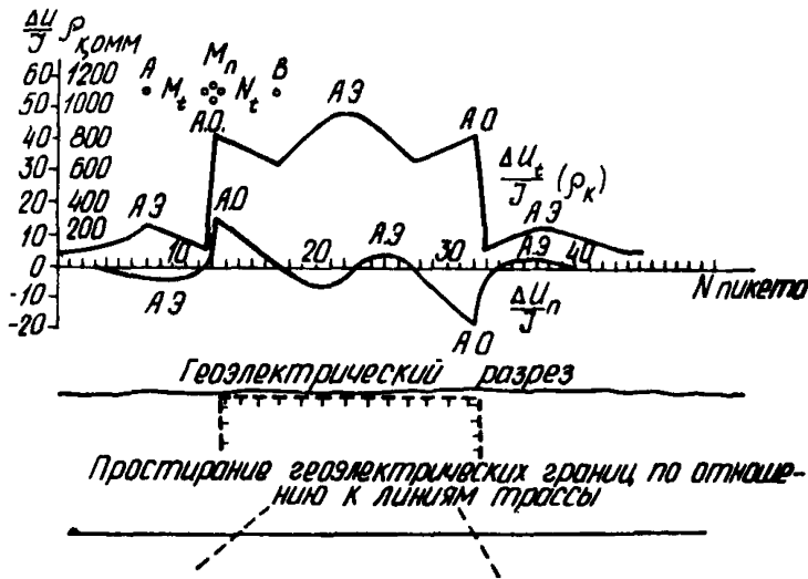
Рис. 3. Графики \frac{\Delta U_{\epsilon}}{\rho} и \frac{\Delta U_{\pi}}{\rho} профилирования по методу двух составляющих симметричной установкой.
