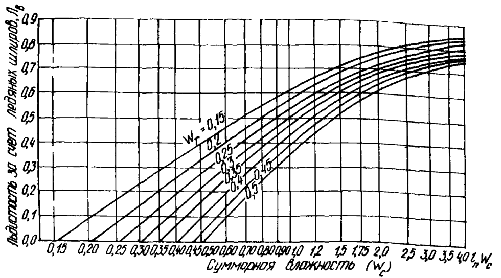
Рис. 1. Номограмма для определения суммарной влажности W_c за счет объемной льдистости L_b и влажности минеральных прослоев W_r
