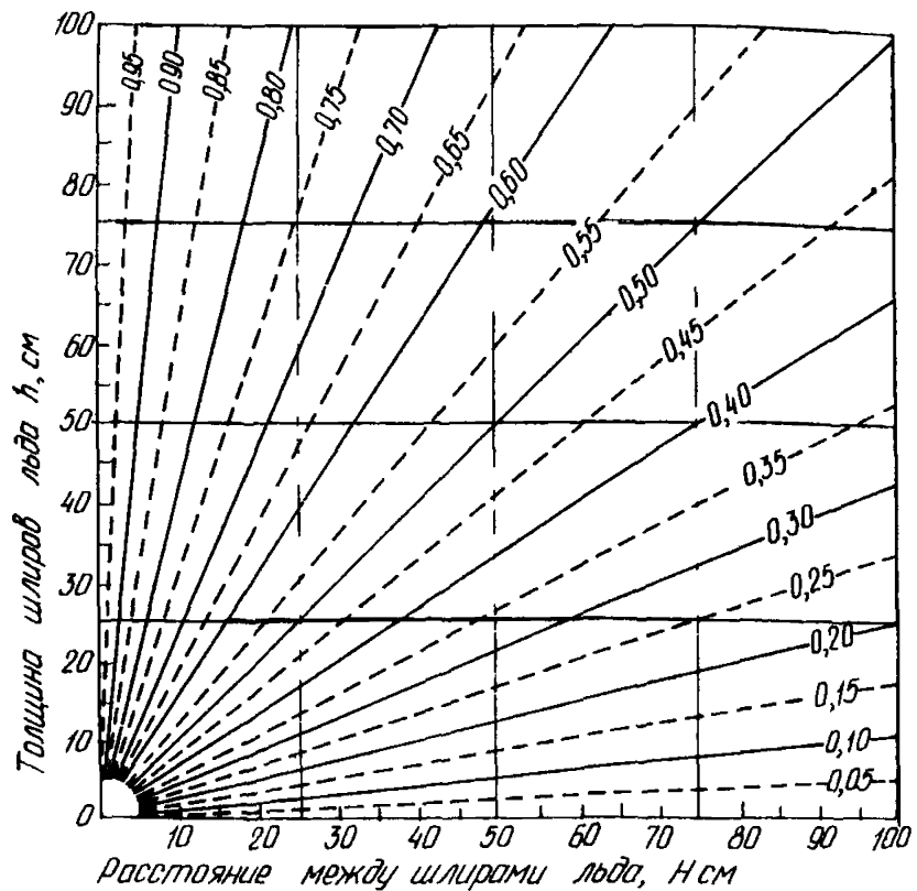
Рис. 2 Номограмма для определения объемной льдистости ( L_b ) мерзлых грунтов со слоистой криогенной текстурой.
