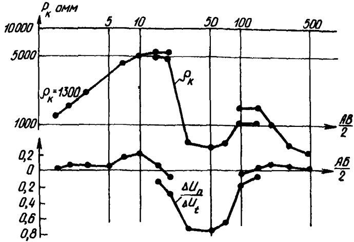
Рис. 1. Кривые \rho_k и \frac{\Delta U_n}{\Delta U_z} симметричного ВЭЗ.
