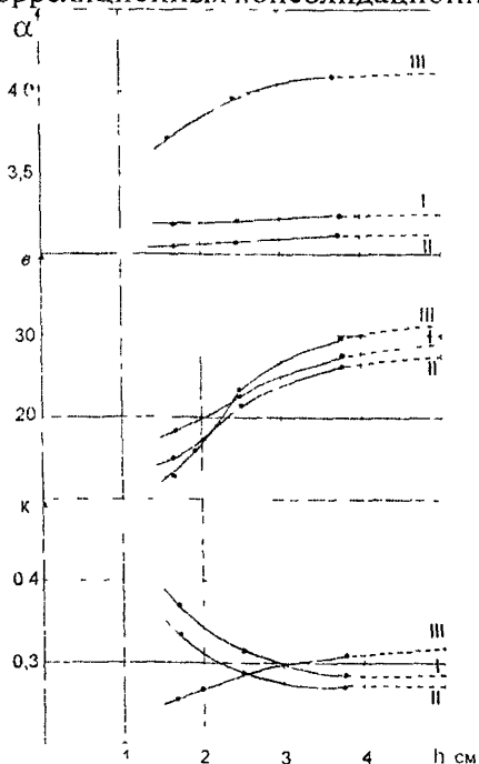
Рис 10. Зависимость a , v , k от высоты образцов торфа. I — Карелия, влажность 600%, II — а/д Кемь-Лоухи, 660%, III — а/д Кривандино-Рошаль, 595%
