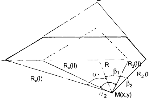
Рис 4 Схема оценки напряженного состояния для нагрузки в виде несимметричной трапеции обшей (I) и дополнительный (II) треугольники
