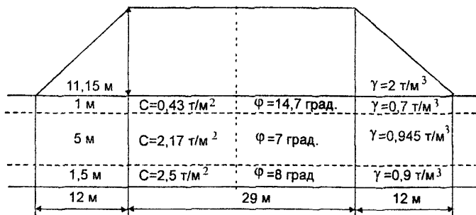
Рис. 6. Схема насыпи на слабом слоистом основании: вариант I – K_{без}=0,56 , S=49,92 см, T=45,96 мес; вариант II – соответственно 0,56, 26,21 см, 3,40 мес
