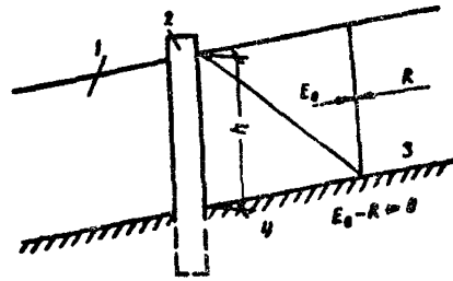
Рис.2. Расчетная схема к проверке свайной удерживающей конструкции на возможность переползания ее грунтом оползневого массива : 1-оползневое тело; 2-свая; 3-поверхность скольжения; 4-коренные породы
