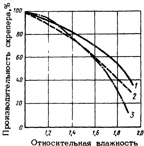
Рис.7. Характер зависимости производительности прицепного скрепера с емкостью ковша 6,0 \text{ м}^3 от влажности грунта: 1–легкая супесь; 2–суглинок; 3–суглинок легкий и тяжелый
