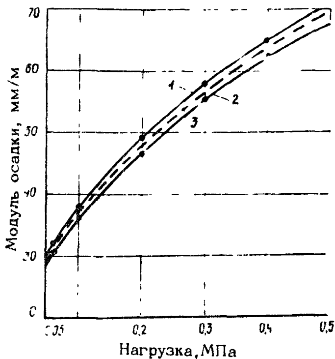
Рис.2. Зависимость модуля осадки от нагрузки: 1,2—опытные кривые; 3—осреднённая кривая
