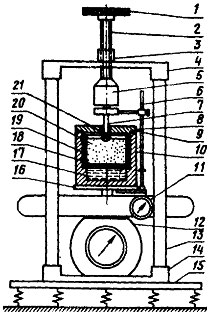
Рис.3. Схема прибора релаксационного типа : 1-ворот; 2-нагрузочный винт; 3-втулка; 4-верхнее основание; 5-шарнирная опора штока; 6-рычажок; 7-шток с шариком; 8-крышка эксикатора; 9-уплотнитель; 10-корпус эксикатора; 11-индикатор смещения шарика; 12-динамометр ДССМ-0,1; 13-стойка; 14-нижнее основание; 15-виброизолирующее основание; 16-площадка для установки образца; 17-вода; 18-диск с отверстиями; 19-металлическое кольцо; 20-образец грунта; 21-сальник
