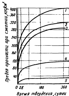
Рис. 2. Изменение активности шлакового вяжущего с различной удельной поверхностью во времени: 1—3000 см²/г; 2—1700 см²/г; 3—1200 см²/г; 4—300 см²/г; 5—100 см²/г
