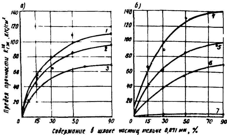
Рис.2. Зависимость предела прочности при сжатии смесей с различным содержанием шлакового вяжущего (а) и цемента (б) от тонкости его измельчения: 1-20% шлака + 2% цемента; 2-10% шлака + 2% цемента; 3-5% шлака + 2% цемента; 4-3% цемента; 5-2% цемента; 6-1% цемента; 7-0% цемента
