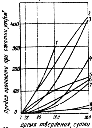
Рис. 2. Изменение активности шлаков разных заводов ( S = 3000 \text{ см}^2/\text{г} ) во времени: 1-константиновского; 2-череповецкого; 3-завода "Азовсталь"; 4-магнитогорского; 5-косогорского; 6-макеевского; 7-новотульского; 8-нижнетагильского; 9-нижнесалдинского
