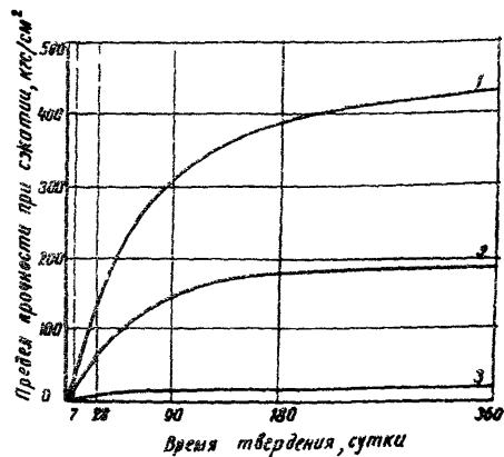
Рис. 2. Изменение активности шлакового вяжущего с различной удельной поверхностью во времени: 1—3000 см 2 /г; 2—1200 см 2 /г; 3—100 см 2 /г (недробленный шлак)
