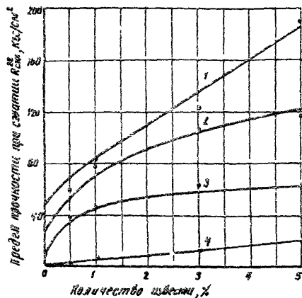
Рис. 1. Влияние содержания извести на активность шлакового вяжущего с различной удельной поверхностью: 1—2000 см 2 /г; 2—1200 см 2 /г; 3—300 см 2 /г; 4—100 см 2 /г (недробленный шлак)
