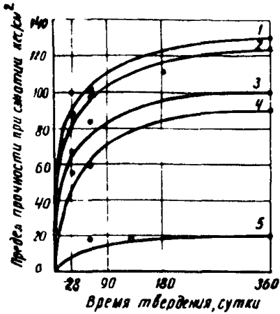
Рис.1. Изменение предела прочности при сжатии смесей с различной удельной поверхностью шлакового вяжущего во времени: 1-3000 см 2 /г; 2-1700 см 2 /г; 3-1200 см 2 /г; 4-300 см 2 /г; 5-100 см 2 /г
