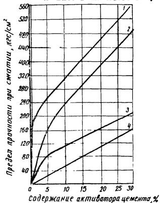
Рис. 1. Влияние содержания цемента на активность шлакового вяжущего с различной удельной поверхностью: 1—3000 см²/г; 2—1700 см²/г; 3—1200 см²/г; 4—300 см²/г; 5—100 см²/г
