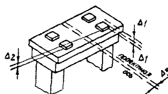
Схема промежуточной опоры
