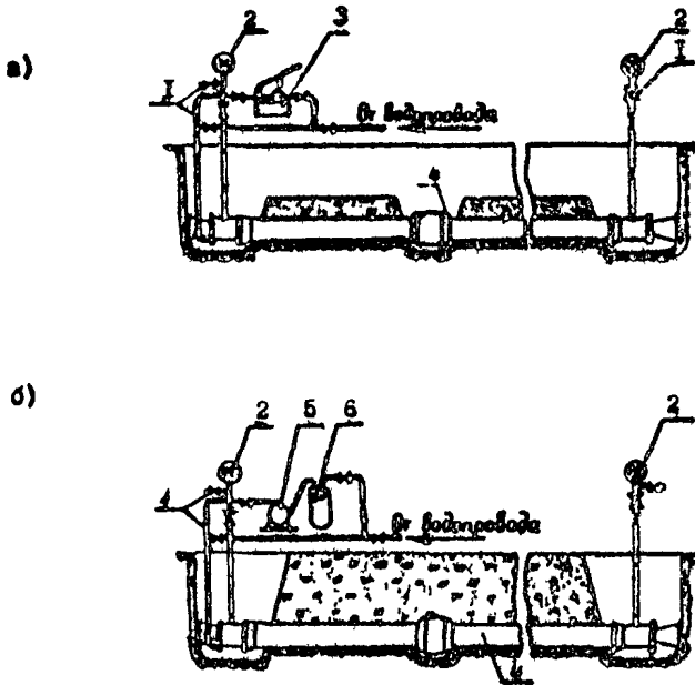
Рис. I Схемы опрессовочных установок
