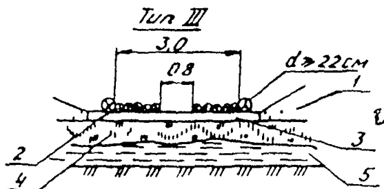
Рис 2 усиление ледовых переправ деревянным настилом
