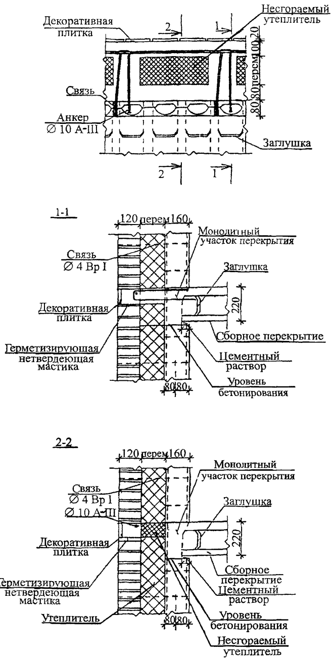
Рисунок 5 – Конструктивное решение облицовки кирпичом сплошных участков наружных стен
