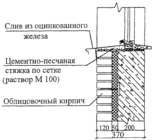
Рисунок 4 – Конструктивное решение облицовки оконных проемов
