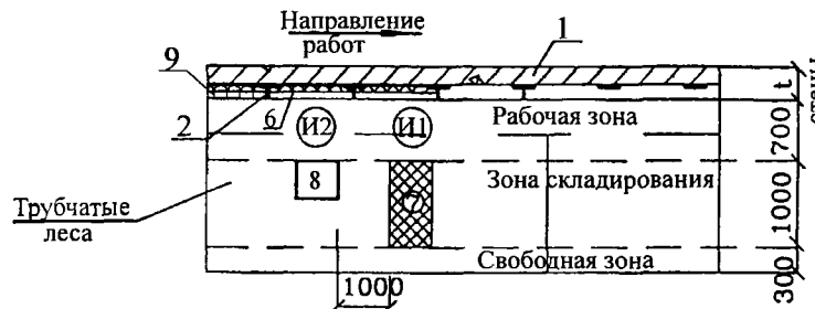
При кирпичной кладке облицовки
