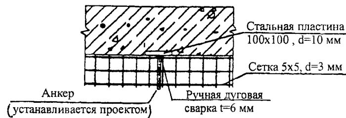
Рисунок 3 – Схема расстановки закладных деталей, устройства металлических анкеров и сеток.
