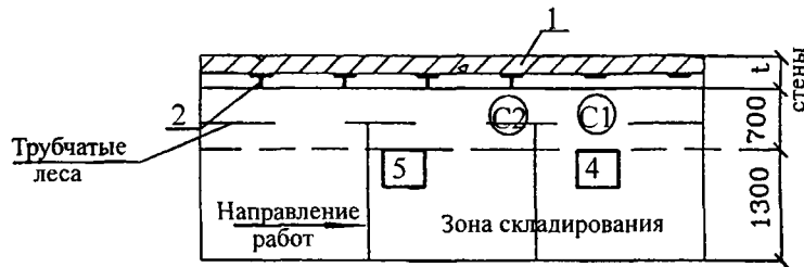
При установке теплоизоляционных плит
