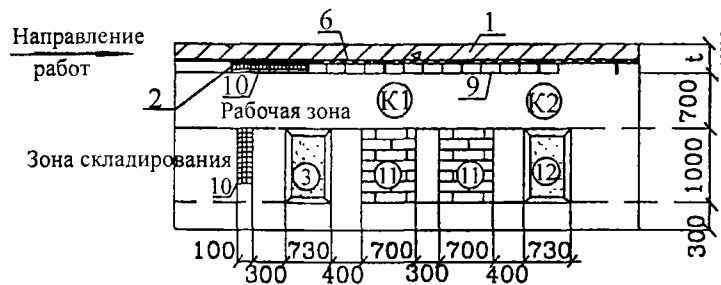
При кирпичной кладке облицовки
