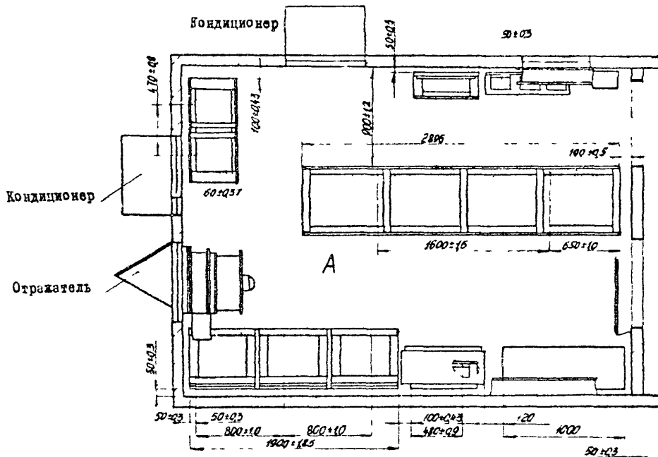
Рис.3. УСТАНОВОЧНЫЙ ПЛАН РАСПОЛОЖЕНИЯ ТЕПЛОТЕХНИЧЕСКОГО ОБОРУДОВАНИЯ В ЭЛЕКТРОСЛОВОМ ОТСЕКЕ А КОНТЕЙНЕРА
