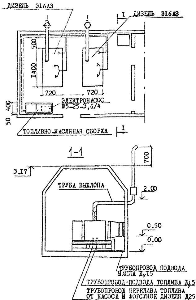
Рис.7. ПЛАН РАЗВОДКИ ТЕХНОЛОГИЧЕСКИХ ТРУБОПРОВОДОВ
