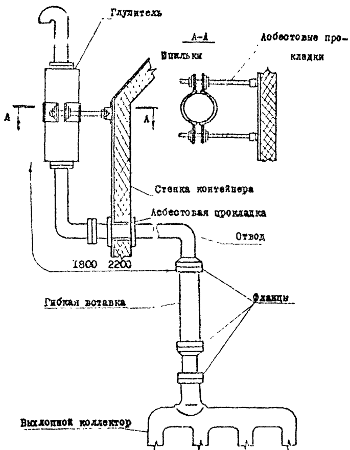
Рис. 8. СХЕМА ВЫХЛОПНОГО ТРУБОПРОВОДА
