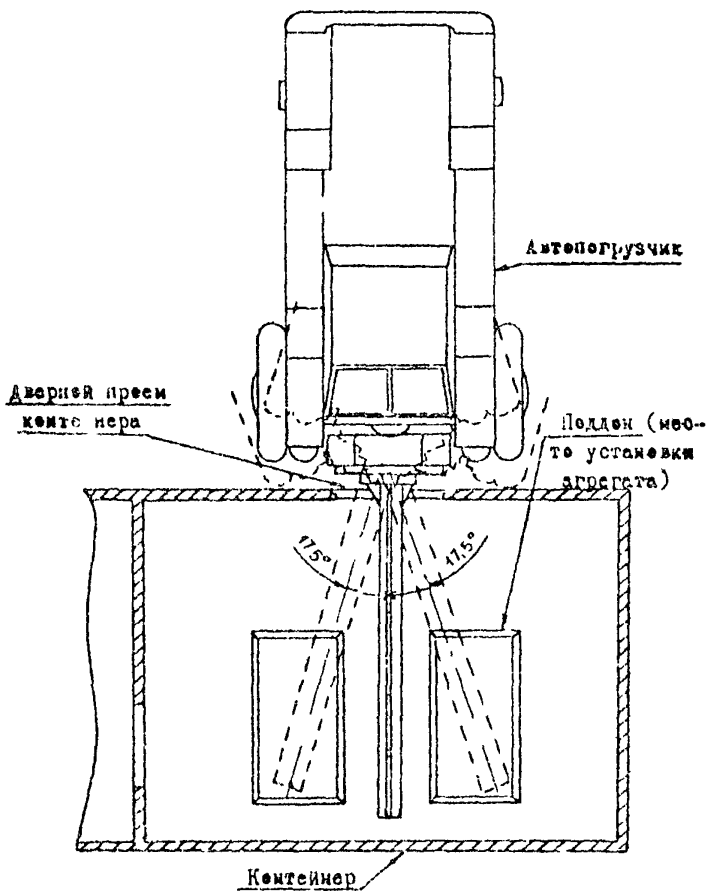
Рис.5. Схема установки дизельного агрегата типа ДГА-16 с помощью автопогрузчика типа 4016 или 4017.
