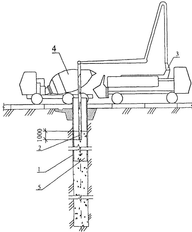
Рисунок 5 – Укладка бетонной смеси в скважину
