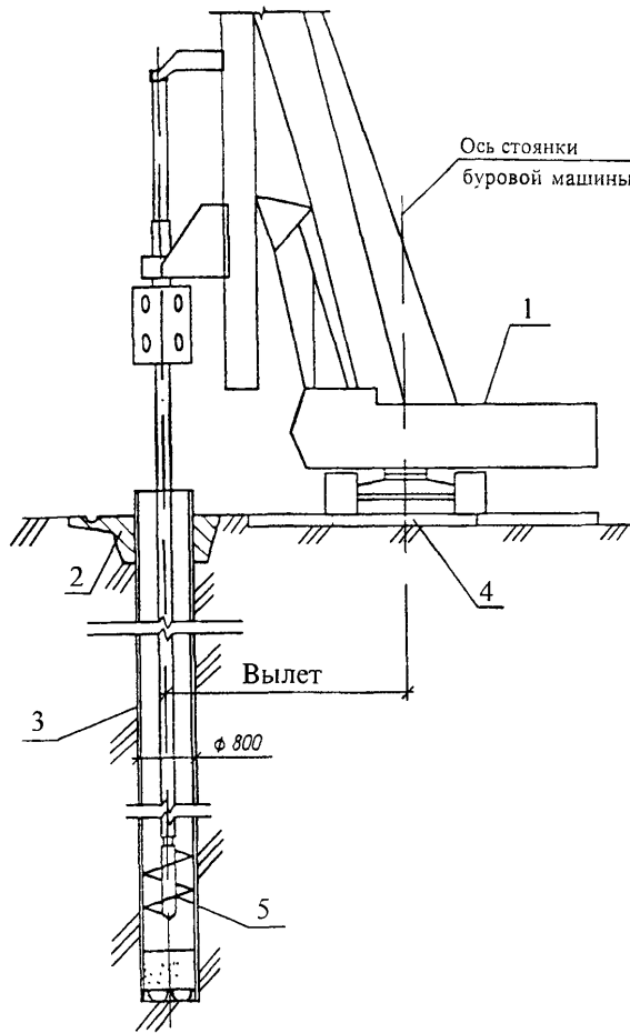
Рисунок 3 – Бурение скважин под защитой обсадной трубы
