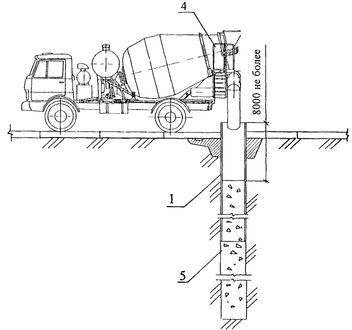
Рисунок 5 – Укладка бетонной смеси в скважину
