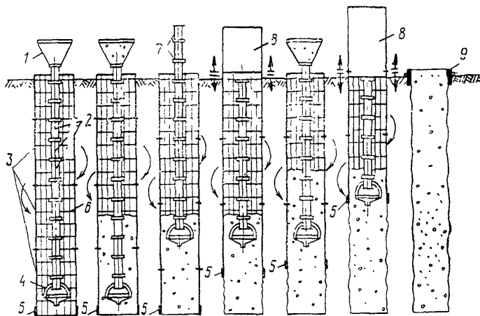
Рисунок 7 – Технологическая схема бетонирования скважины
