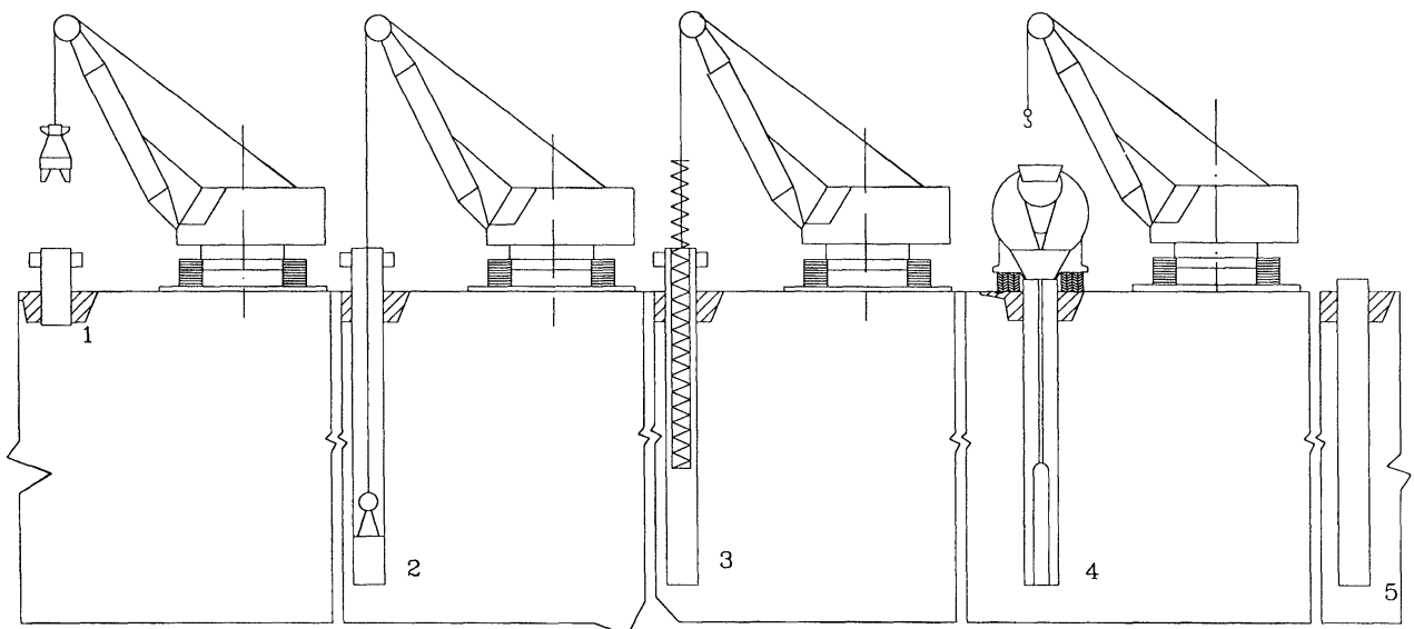
Рисунок 2 - Основные этапы устройства буронабивной сваи
