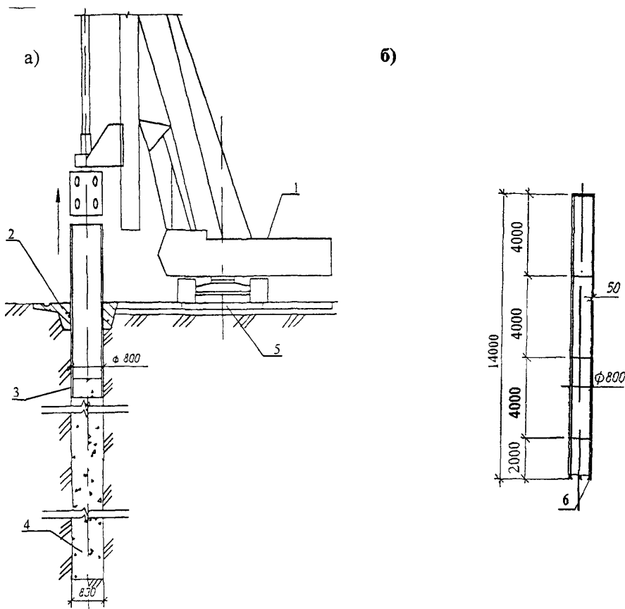
Рисунок 6 – Извлечение обсадной трубы
