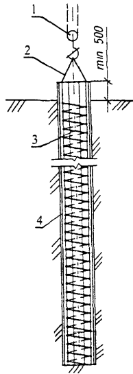
Рисунок 4 – Установка арматурного каркаса сваи
