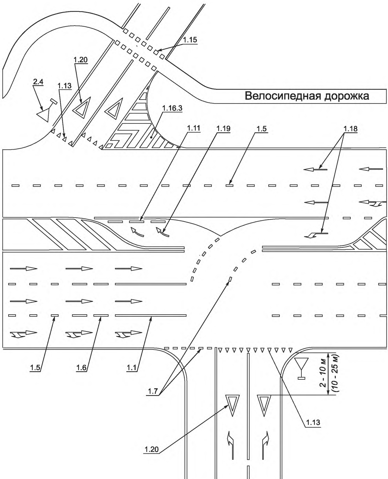
Рисунок В.10 — Пример нанесения разметки канализованного пересечения
