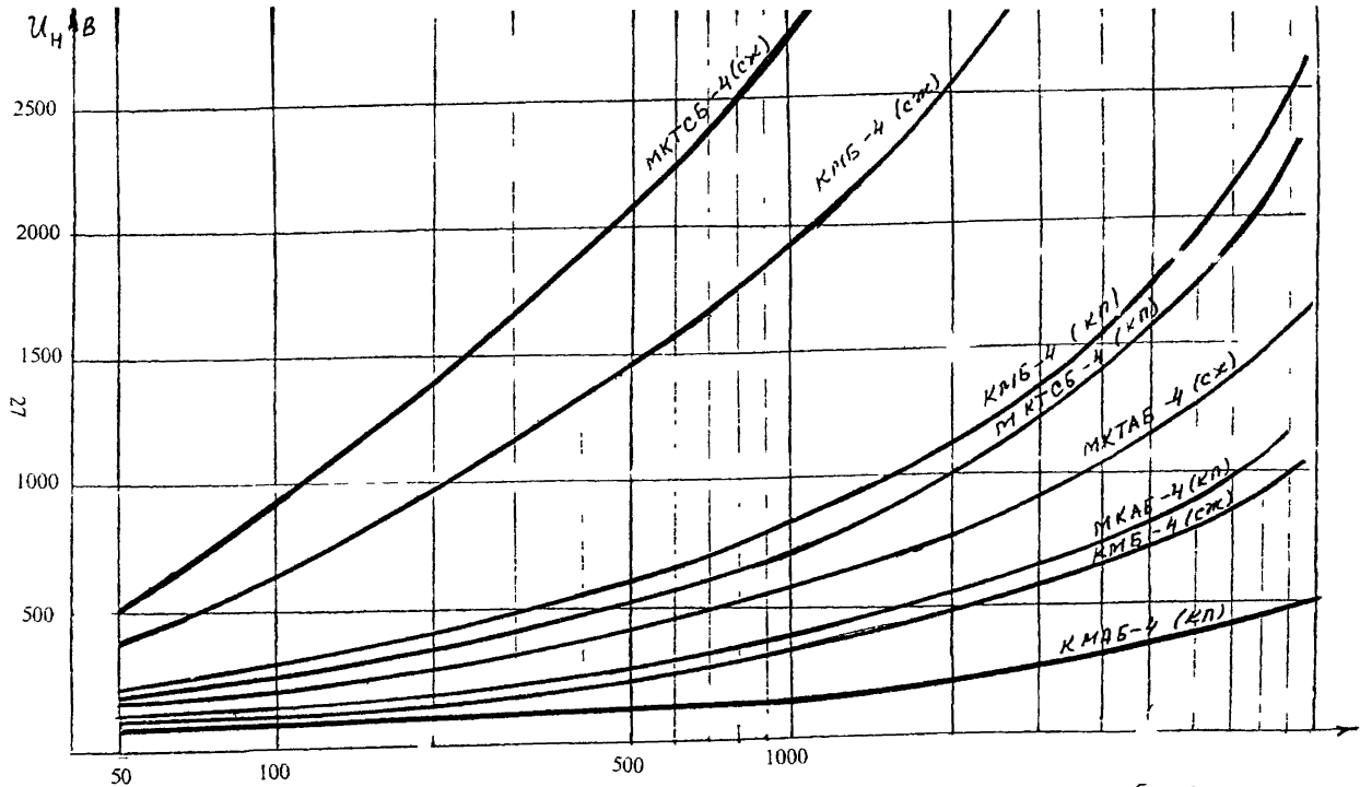
Рис 2 Расчетные величины наводимых напряжений в кабелях в зависимости от удельного сопротивления земли
