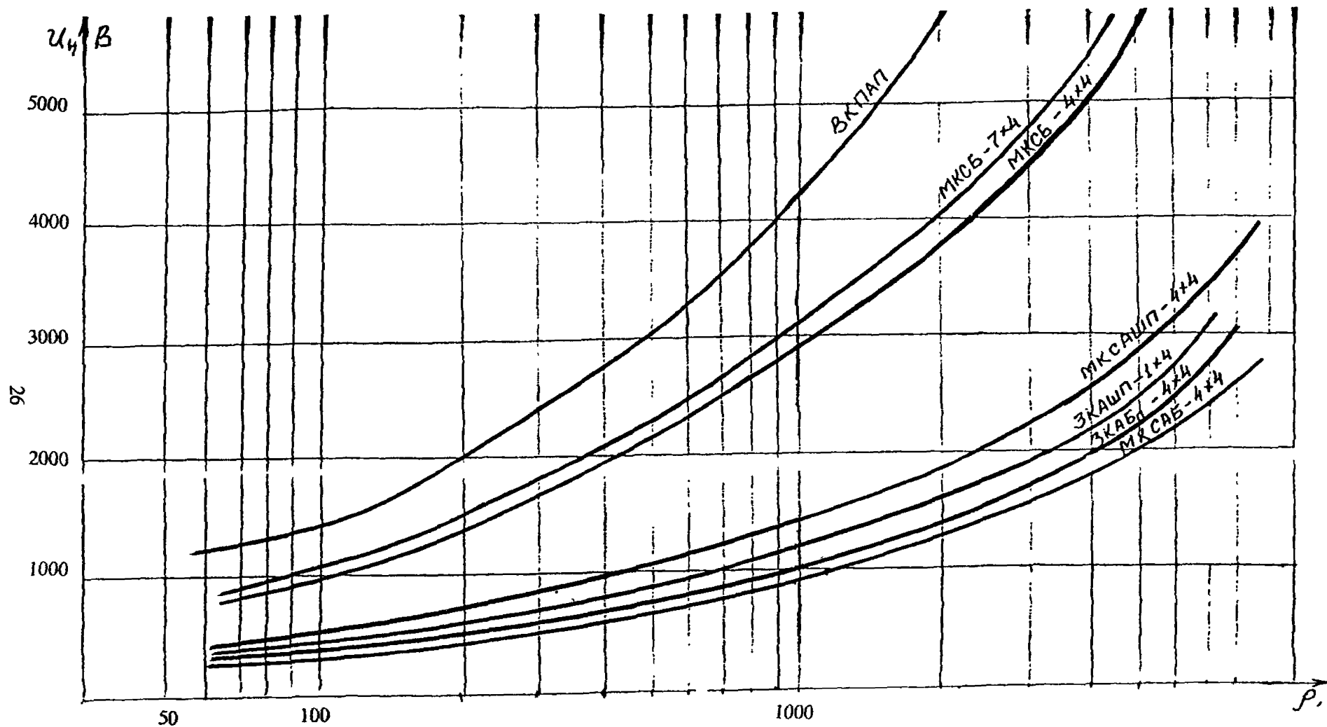
Рис.1 Расчетные величины наводимых напряжений в кабелях в зависимости от удельного сопротивления земли
