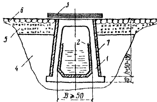
рис. 4. Поперечный разрез по левостороннему лотку:
