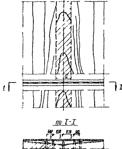
Рис. 13. Свободный пропуск наледи (к примеру 9): а - ширина наледи в бытовых условиях
