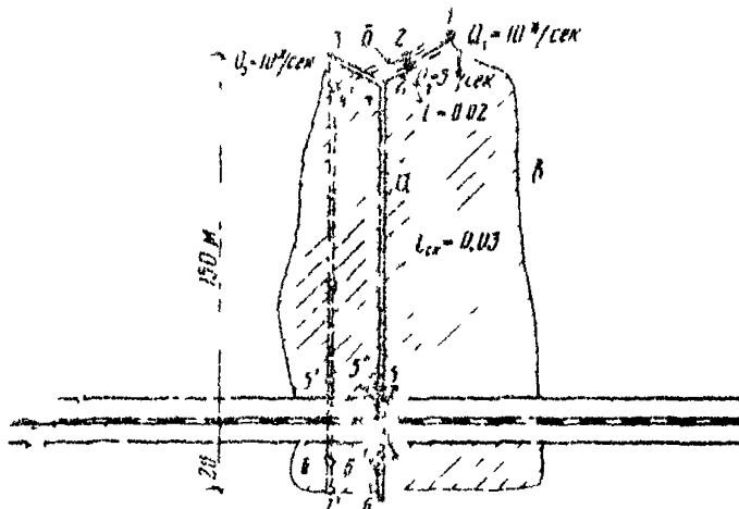
Рис. 5. Схема противоаварийных мероприятий (к примеру 4). а - утепленный лоток; б - дренаж; в - контуры наледи в зимний период
