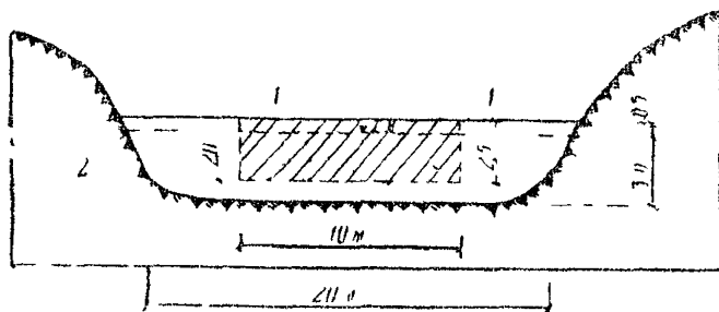
Рис. 7. Поперечный разрез лога (к примеру 5): 1 - контур фундамента оголовка МБПТ; 2 - водоупорный грунт
