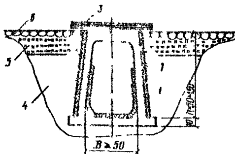
Рис. 1. Поперечный разрез по железобетонному лотку.
