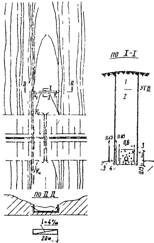
Рис. 8. Схема противоналедных сооружений (к примеру 5): 1 - местный грунт; 2 - крупный песок; 3 - щебень; 4 - щит; 5 - экран из глины; К - смотровые колодцы
