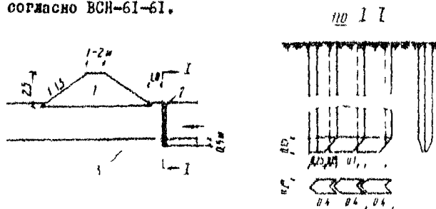
Рис. 12. Схема экраняющей стенки с земляным удерживающим валом:
