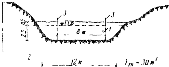
Рис. 11. Поперечный разрез лога (к примеру 8): 1 - песок с гравием; 2 - аргиллиты; 3 - контур фундамента оголовка БПТ
