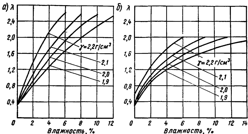
Рис. 20. Графики для определения коэффициентов теплопроводности гравийно-песчаных смесей:
