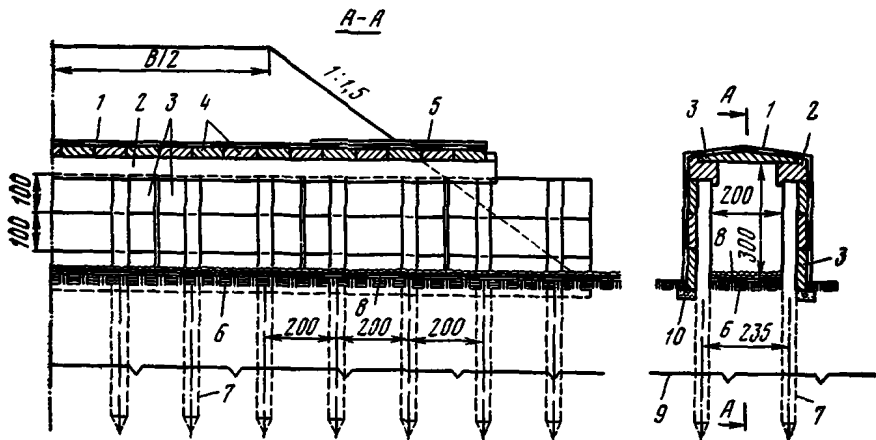
Рис. 7. Конструкция прямоугольной железобетонной свайно-щитовой трубы Ленгипротранса:
