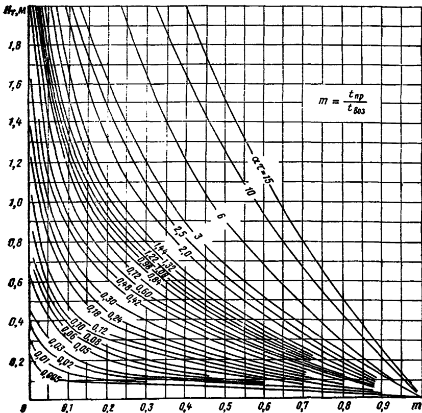
Рис. 12. Зависимость между толщиной слоя теплоизоляции H_T и коэффициентом m
