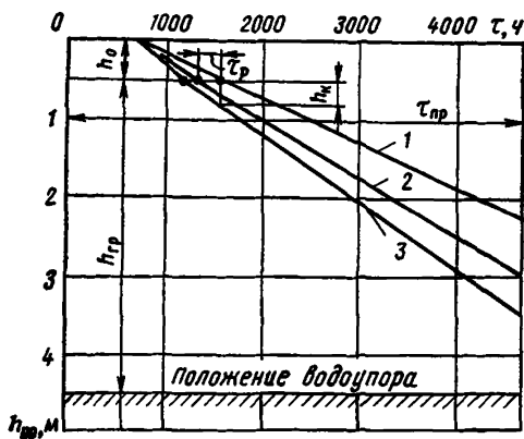
Рис. 17. Ход промерзания поверхностного и подруслового потоков:
