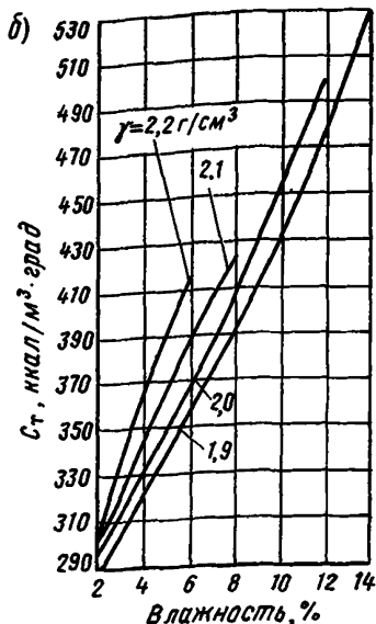
Рис. 21 Графики для определения объемной теплоемкости гравийно-песчаных смесей:
