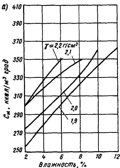
Рис. 21 Графики для определения объемной теплоемкости гравийно-песчаных смесей:
