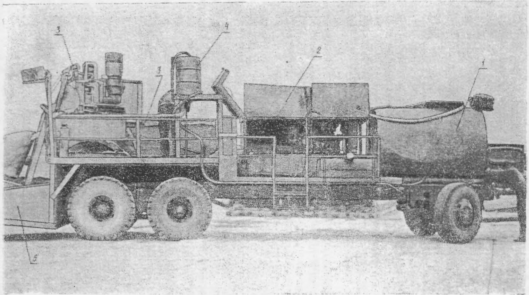
Рис. 3. Заливщик швов:
