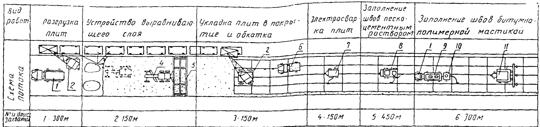
Рис. 1. Технологическая схема устройства сборного покрытия:
