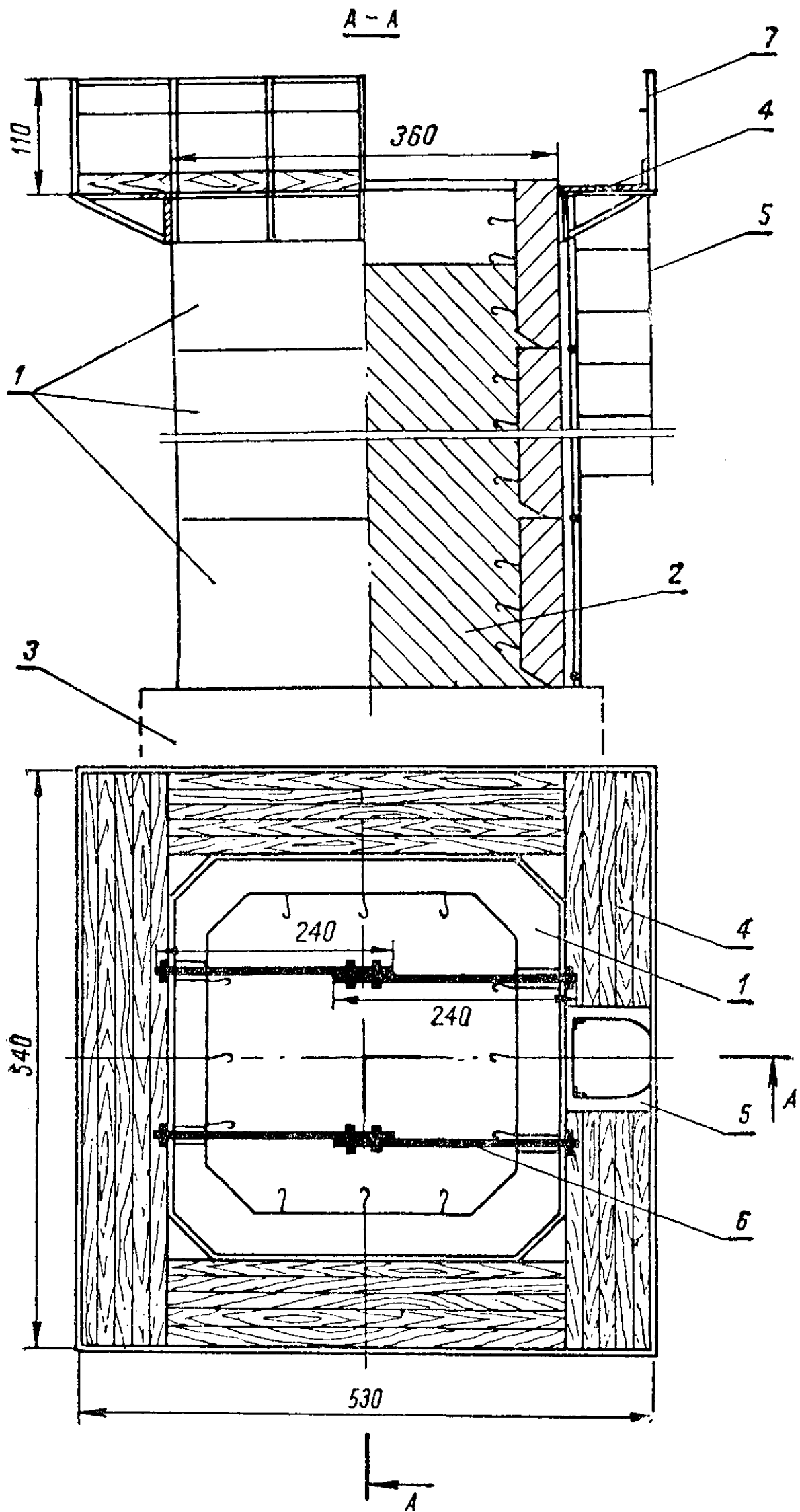
Рис. 4. Подвесные подмости:
