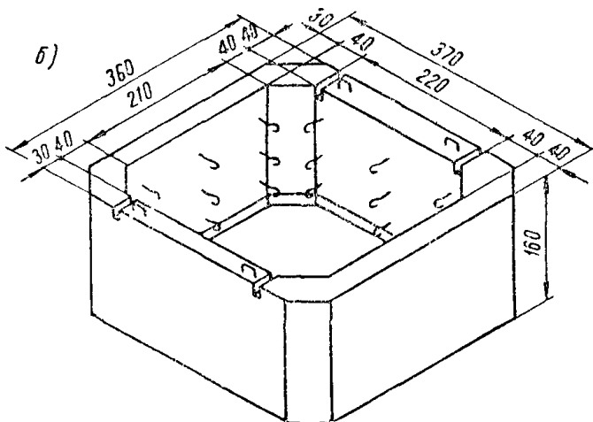
Рис. 2. Элементы сборной опоры: а—сборный подферменник; б—контурный блок
