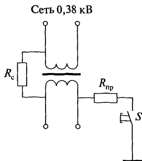
Рис. П.6.2. Схема соединения однофазных трансформаторов
