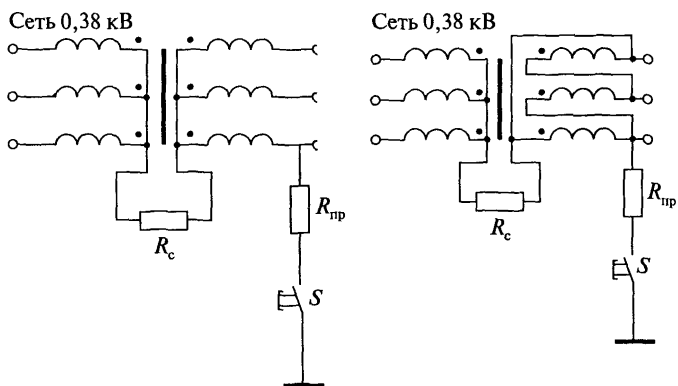
Рис. П.6.1. Схема соединения трехфазных трансформаторов
