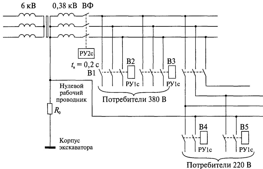
Рис. П.3.1. Схема размещения двухступенчатой защиты от утечек тока во внутриэкскаваторной сети 220–380 В:
