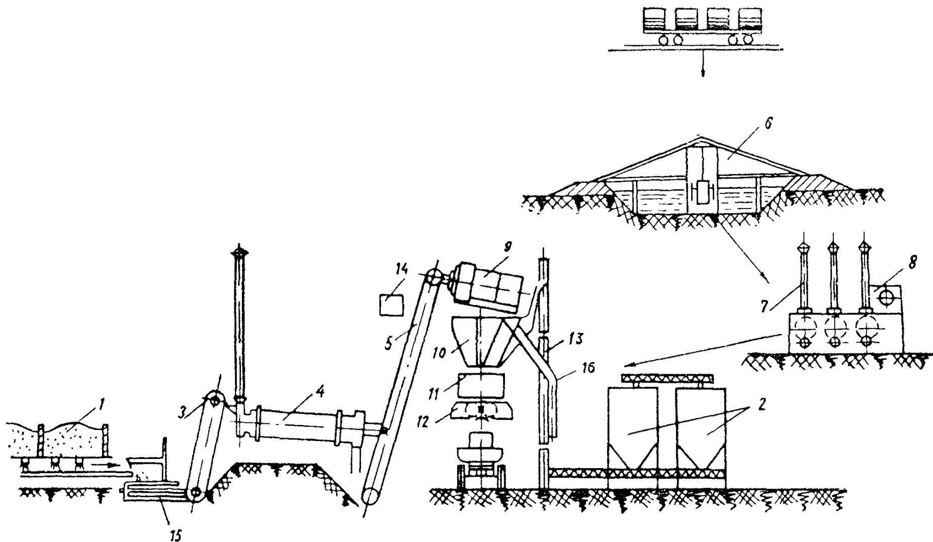
Технологическая схема АБЗ со смесителями Д-325 (Д-152):
