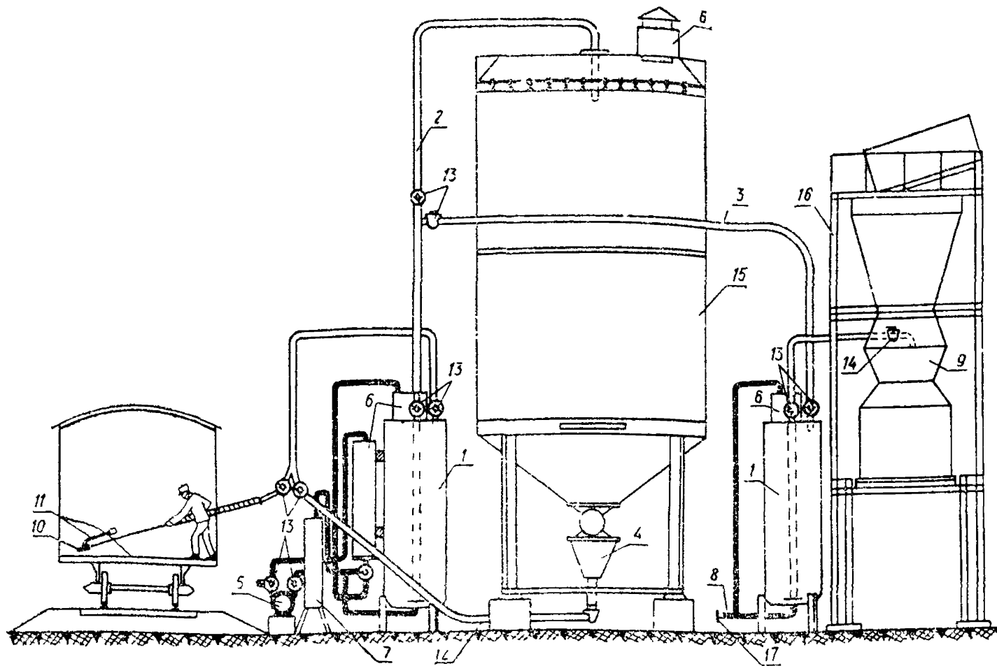
Рис 2 Технологическая схема работы монжусов на АБЗ.
