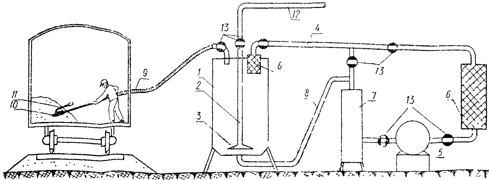
Рис 1 Схема работы монжуса при выгрузке минерального порошка из железнодорожного вагона и подача его на склад:
