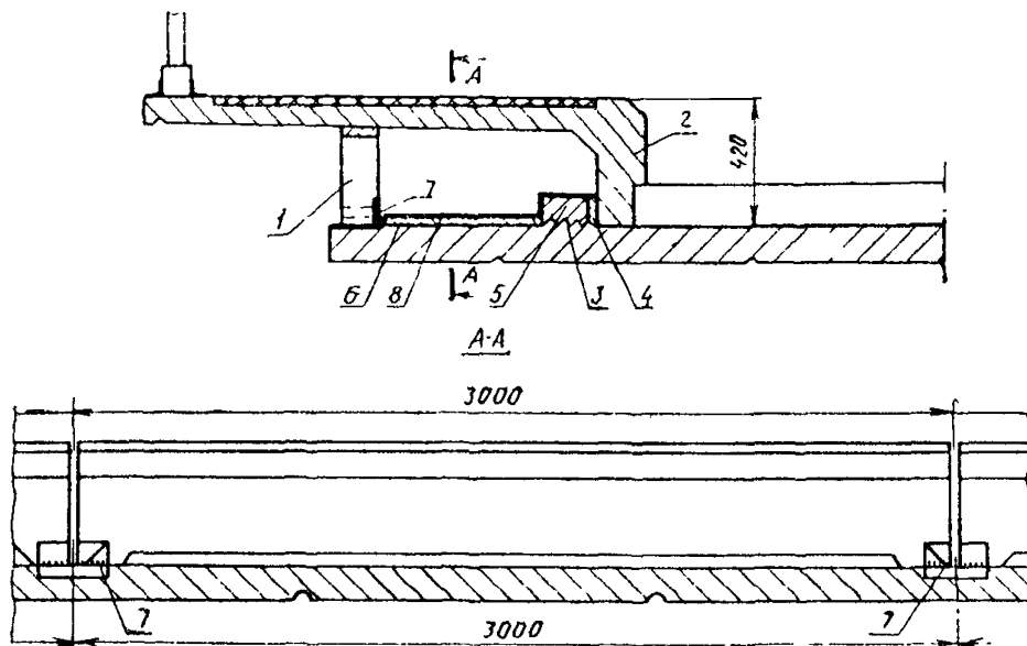
Рис. 1. Конструкция тротуаров
