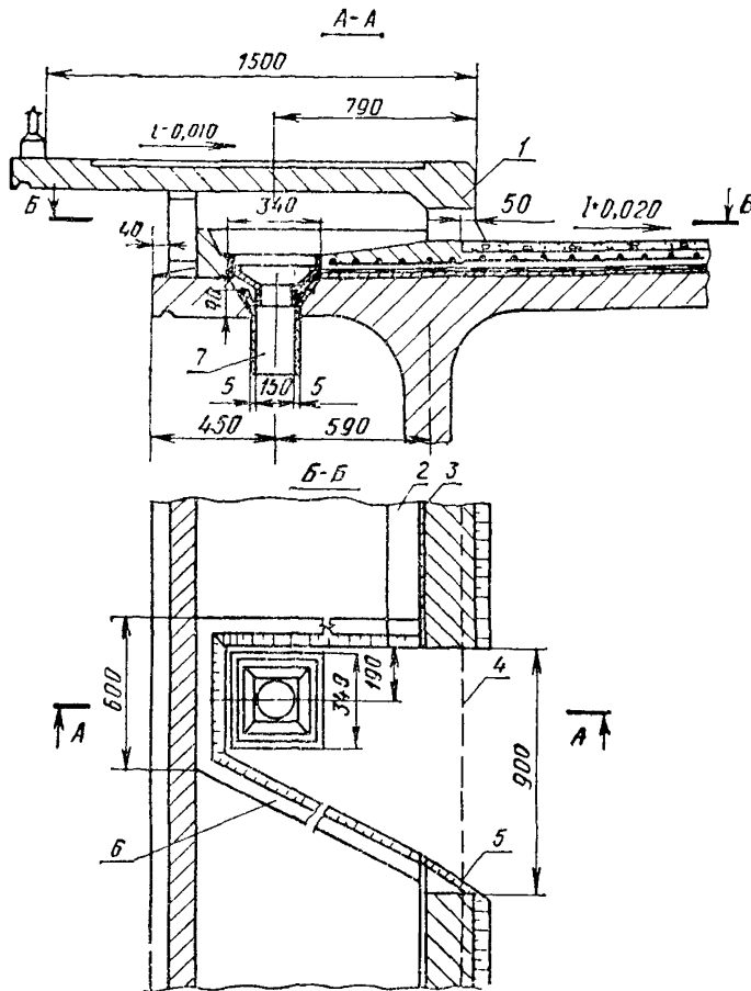
Рис 2. Устройство водоотвода:
