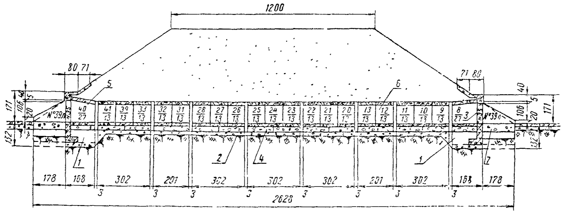
Рис 4. Конструкция и последовательность монтажа элементов трубы:
