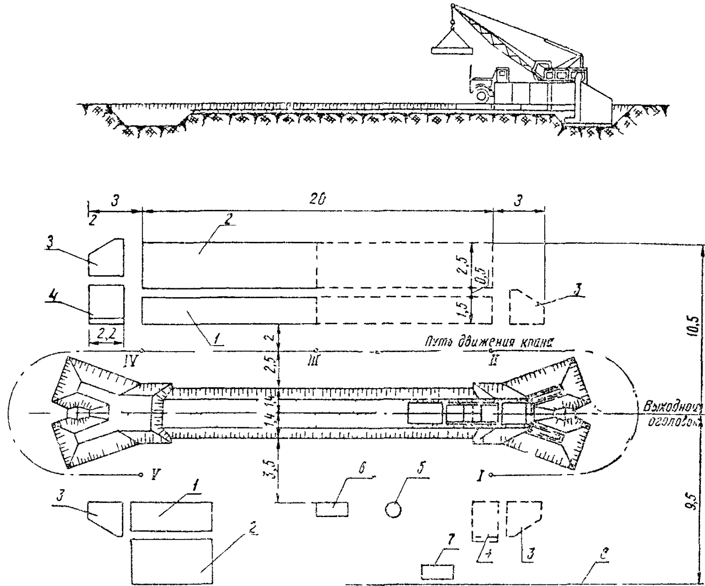
Рис 3 План строительной площадки
