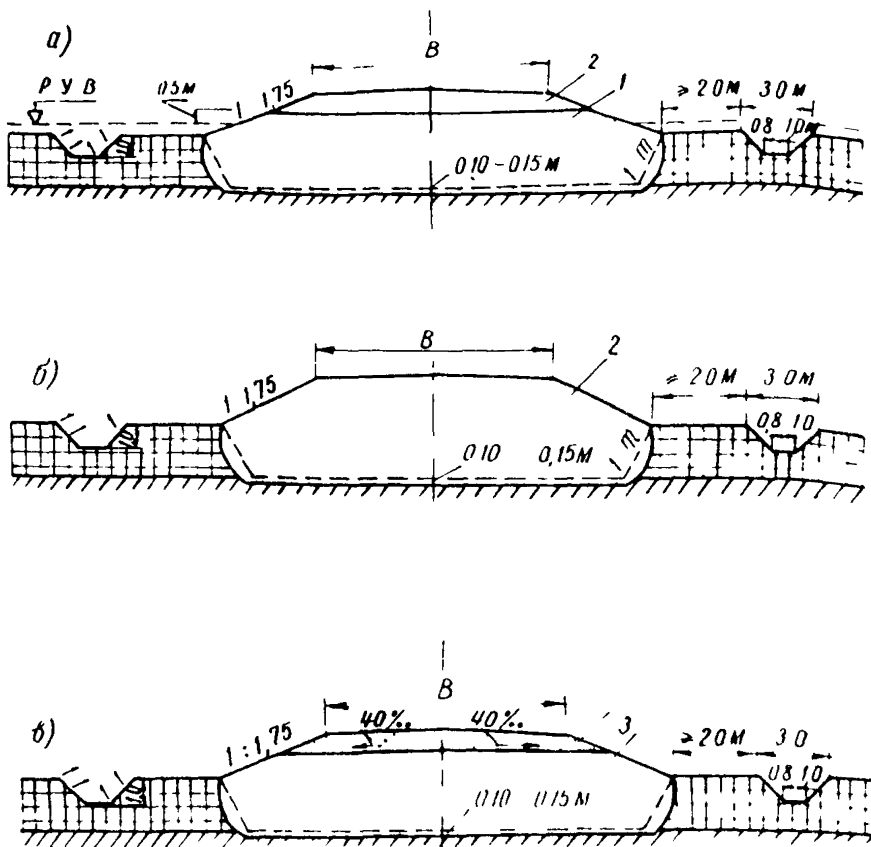
Рис.1. Конструкции земляного полотна с полным выторфовыванием на болотах 1 типа
