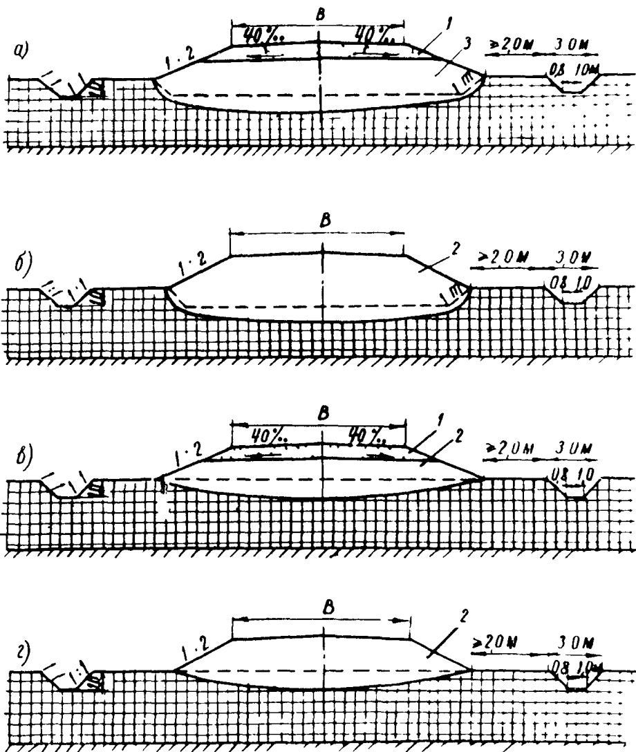
Рис.3. Конструкции земляного полотна с частичным (а б) и полным (в, г) использованием торфа в основании насыпей : 1-песчаный и легкий супесчаный грунт; 2-глинистый грунт ; 3-пылеватый глинистый грунт
