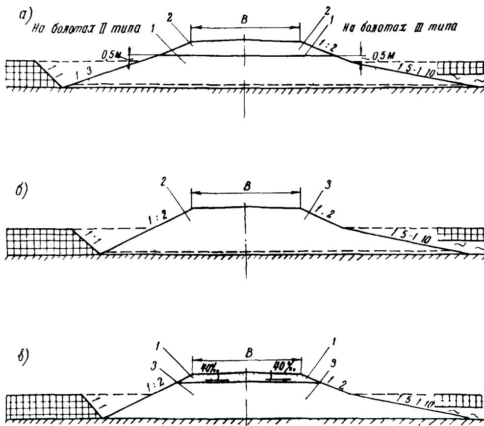
Рис.2. Конструкция земляного полотна с полным выторфовыванием на болотах II и III типов: 1-песчаный и легкий супесчаный грунт; 2-глинистый грунт 3-пылеватый глинистый грунт
