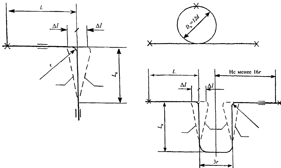
Рисунок Д.1 — Расчетные схемы гнутых компенсаторов
