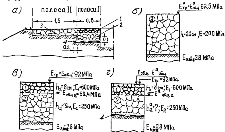
Рис.1. 1 - щебень I-го класса, пропитанный битумом; 2 - щебень I-го класса; 3 - местный несортированный щебень
