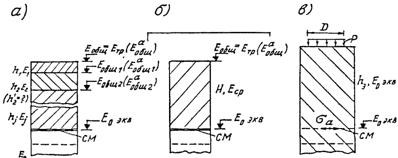
Рис.2. Схемы к расчету конструкций укрепления обочин
