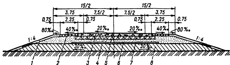
Рис. 9. Поперечный профиль дорожной конструкции типа С:
