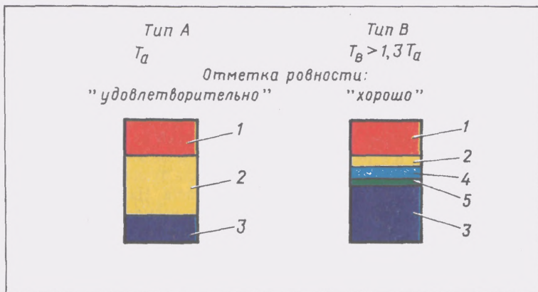
Рис. 6. Показатели долговечности и ровности покрытия при устройстве традиционной конструкции дорожной одежды (тип А) и дорожной одежды с пенопластом (тип В): 1 — покрытие и основание дорожной одежды; 2 — песок; 3 — грунт; 4 — пенопласт Styrofoam; 5 — геотекстиль
