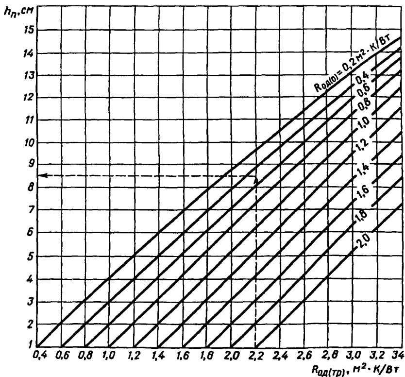
Рис. 12. График для определения необходимой толщины слоя пенопласта Styrofoam: R_{од(тр)} — требуемое термическое сопротивление дорожной одежды; R_{од(доп)} — термическое сопротивление дорожной одежды без слоя пенопласта
