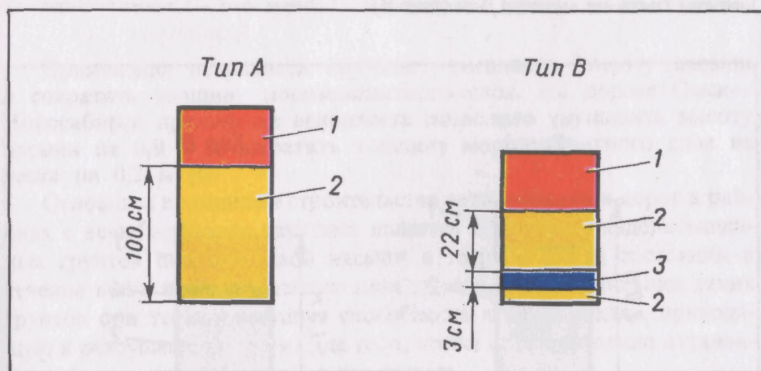
Рис. 1. Конструкции дорожной одежды равноценные по морозоустойчивости в условиях Москвы:
