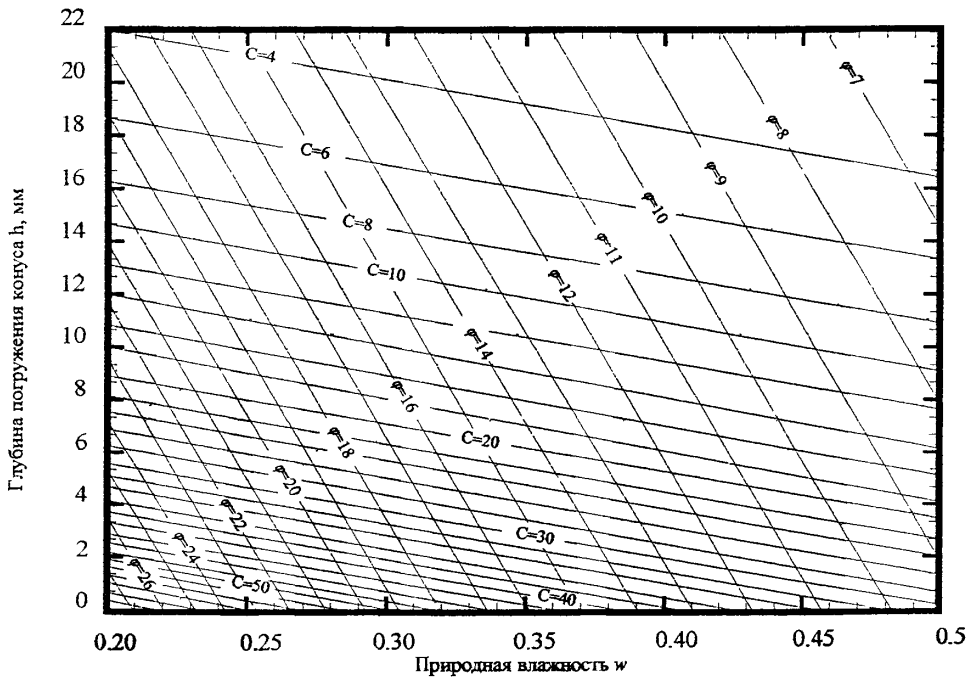
Рисунок Е.6 – Номограмма для определения удельного сцепления c_n , кПа, и угла внутреннего трения \varphi , град., озерно-морских и озерно-ледниковых глинистых грунтов
