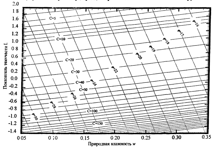
Рисунок Е.2 – Номограмма для определения сцепления c_u , кПа и угла внутреннего трения \varphi_u , град., ледниковых (моренных) глинистых грунтов
