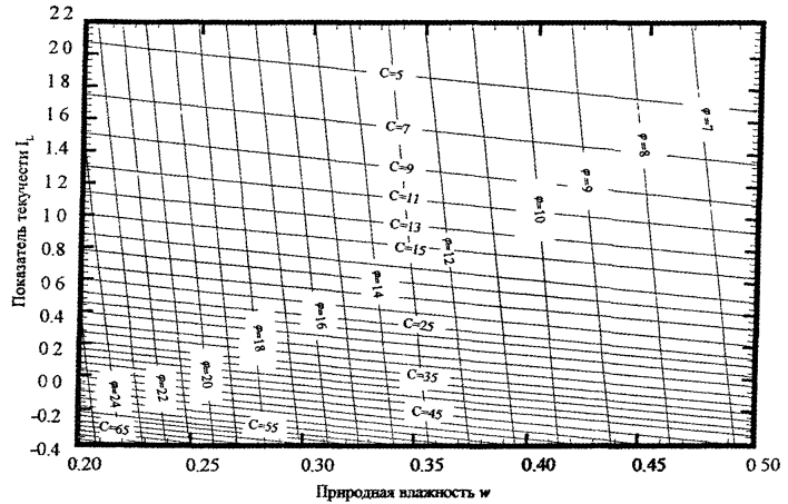
Рисунок Е.1 – Номограмма для определения удельного сцепления c_u , кПа и угла внутреннего трения \varphi_u , град., озерно-ледниковых глинистых грунтов
