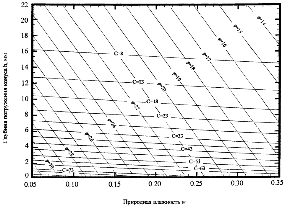
Рисунок Е.7 – Номограмма для определения удельного сцепления c_n , кПа, и угла внутреннего трения \varphi , град., ледниковых (моренных) глинистых грунтов
