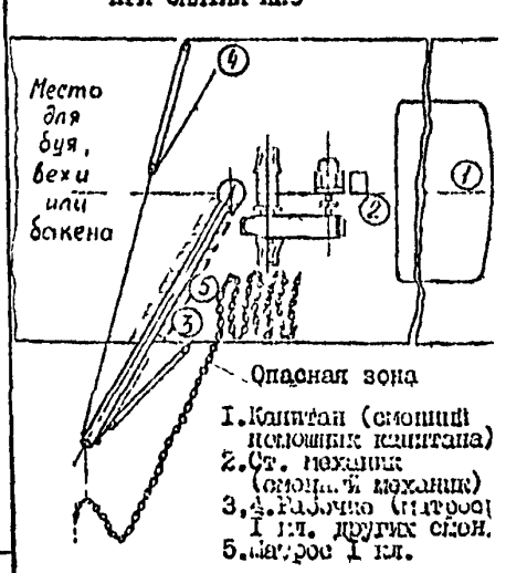
СХЕМА РАССТАНОВКИ ИСПОЛНИТЕЛЕЙ ПРИ СНЯТИИ ШЗ
